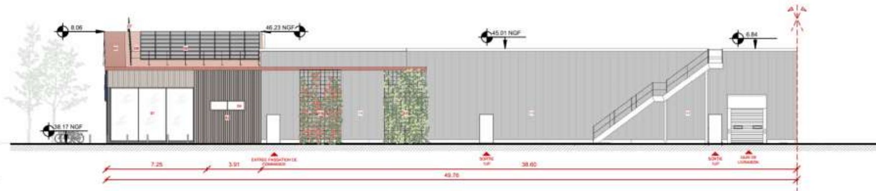
FACADE NORD PROJET
