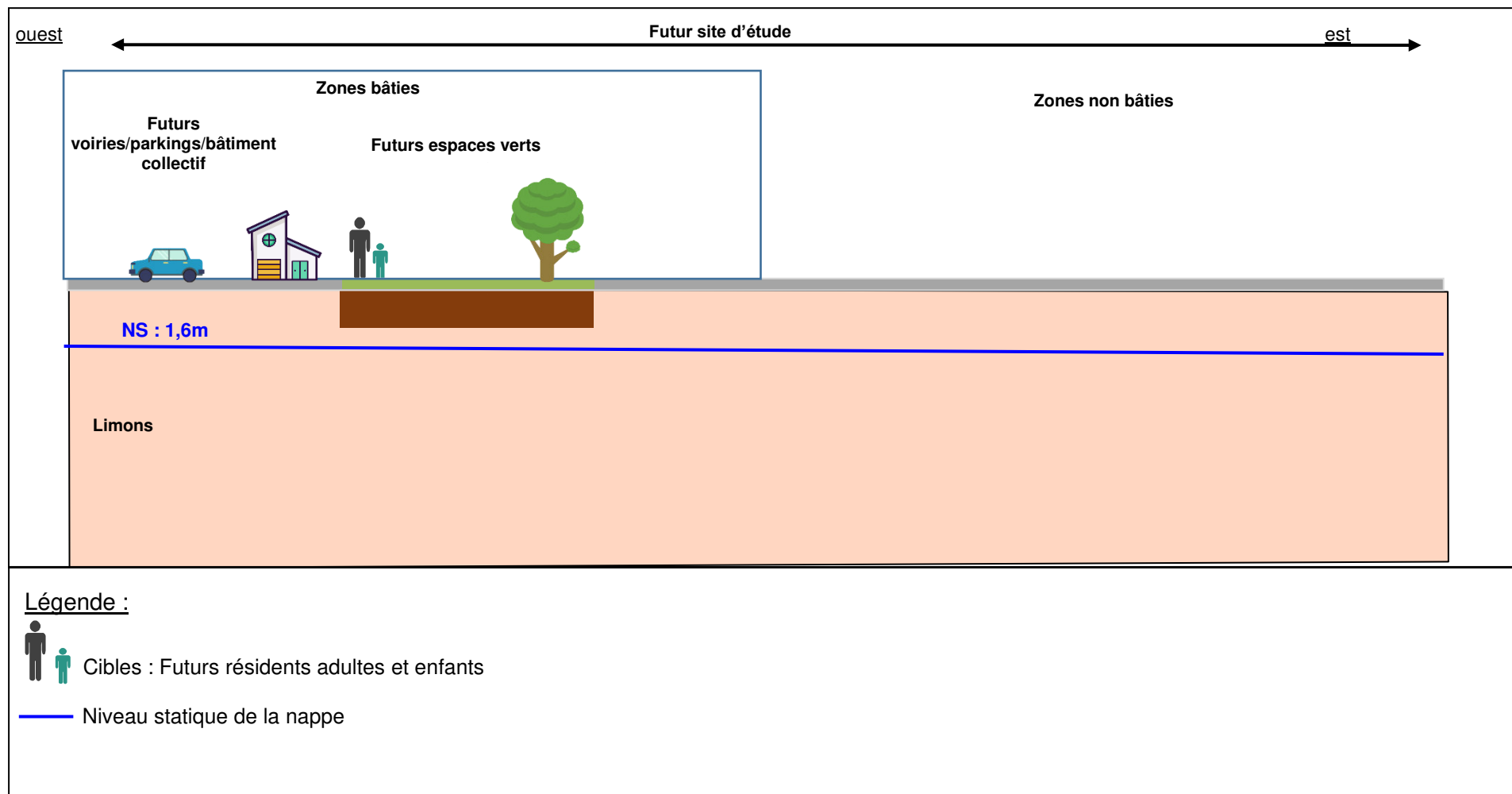
Figure 6. Schéma conceptuel du site - usage futur (sensible)
