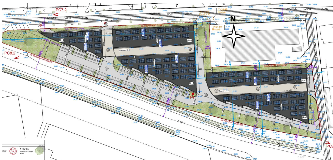
Figure 5 : Plan de composition et aménagement paysager – AVP Source : INNOVINFR
