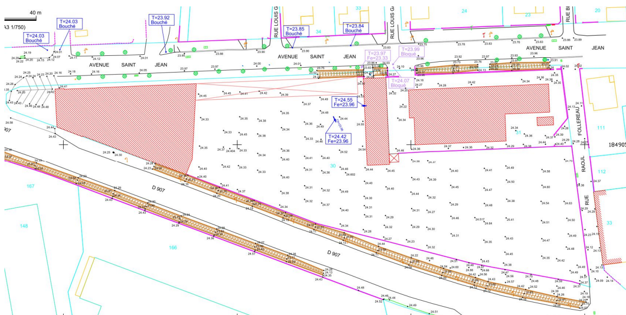
Figure 8 : Topographie au droit de la parcelle étudiée Source : Géomètre
