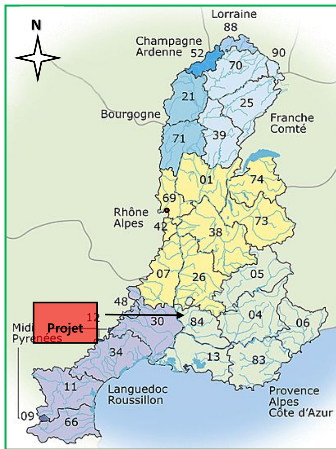
Figure 21 : Carte du SDAGE du bassin Rhône-Méditerranée Source : Gest'Eau.fr
