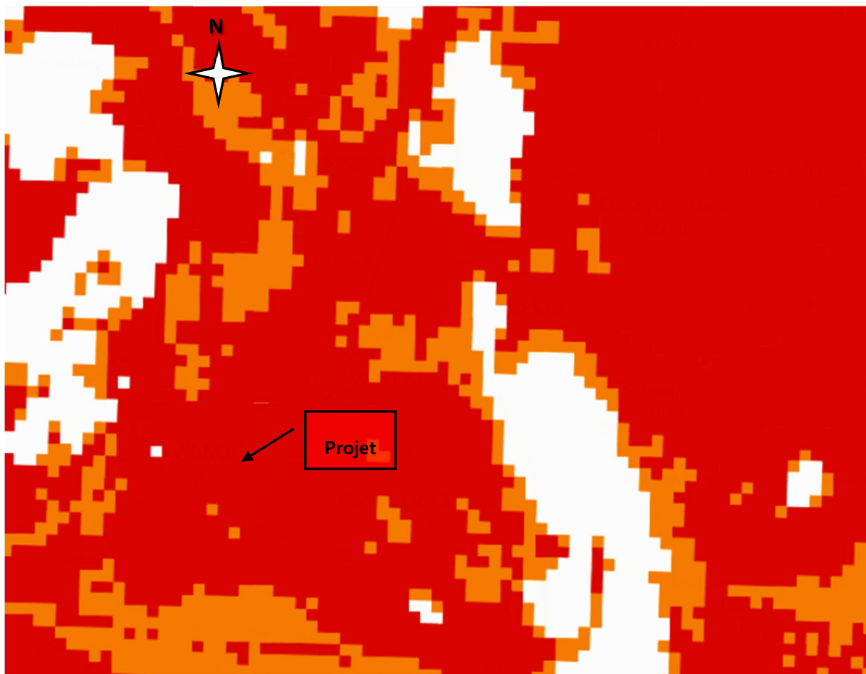
Figure 16 : Carte de sensibilité vis-à-vis des remontées de nappes Source : BRGM
