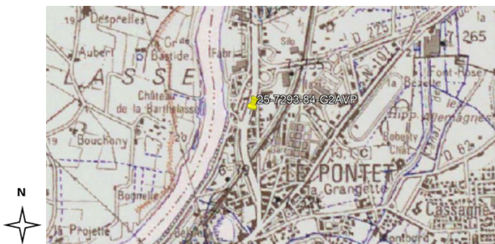
Figure 10 : Carte géologique de au 1/50 000 Source : BRGM
