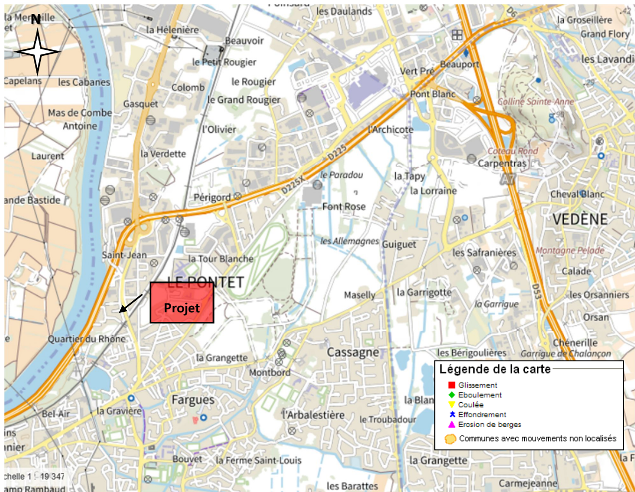
Figure 17 : Carte des mouvements de terrain Source : BRGM
