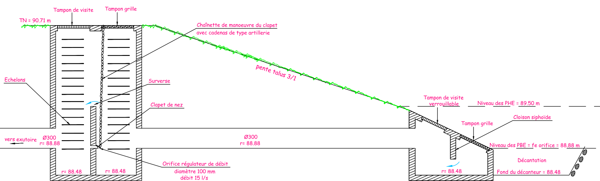
COUPE TRANSVERSALE (Sans Echelle)
