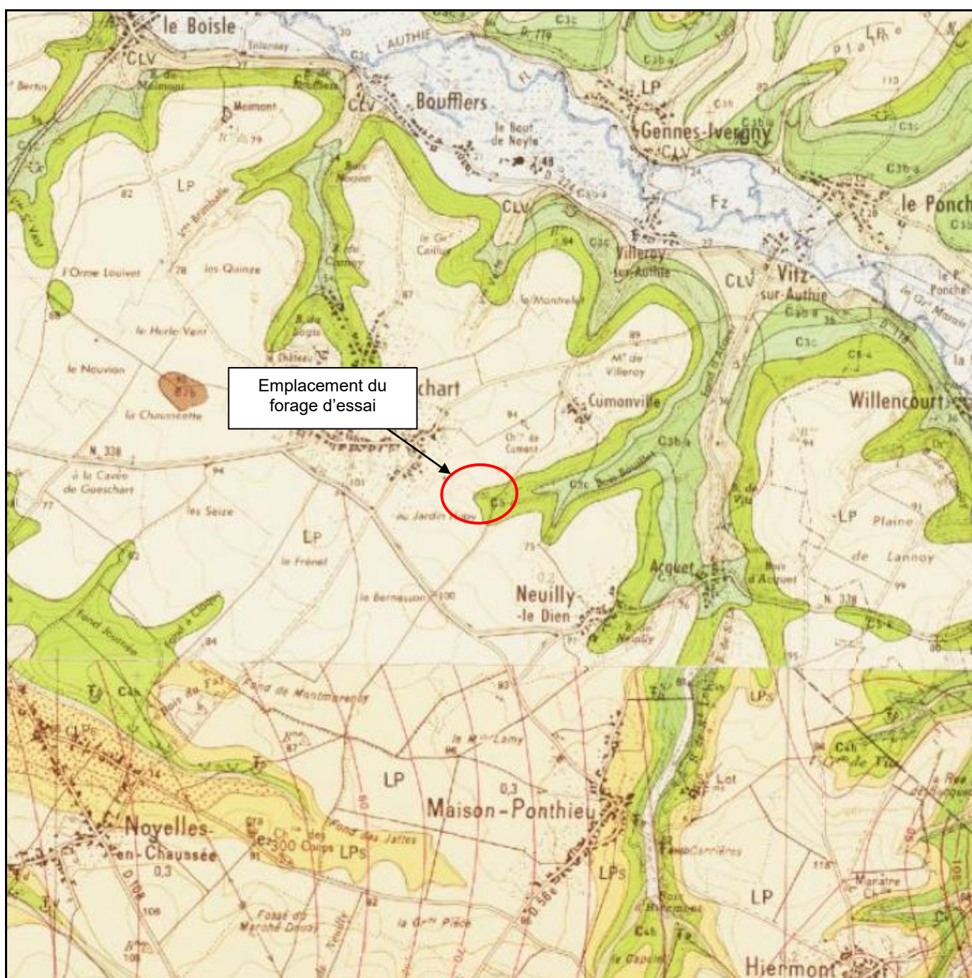
Figure 6 : Extrait de la carte géologique d'ABBEVILLE et de HESDIN (1/50 000 ème )
