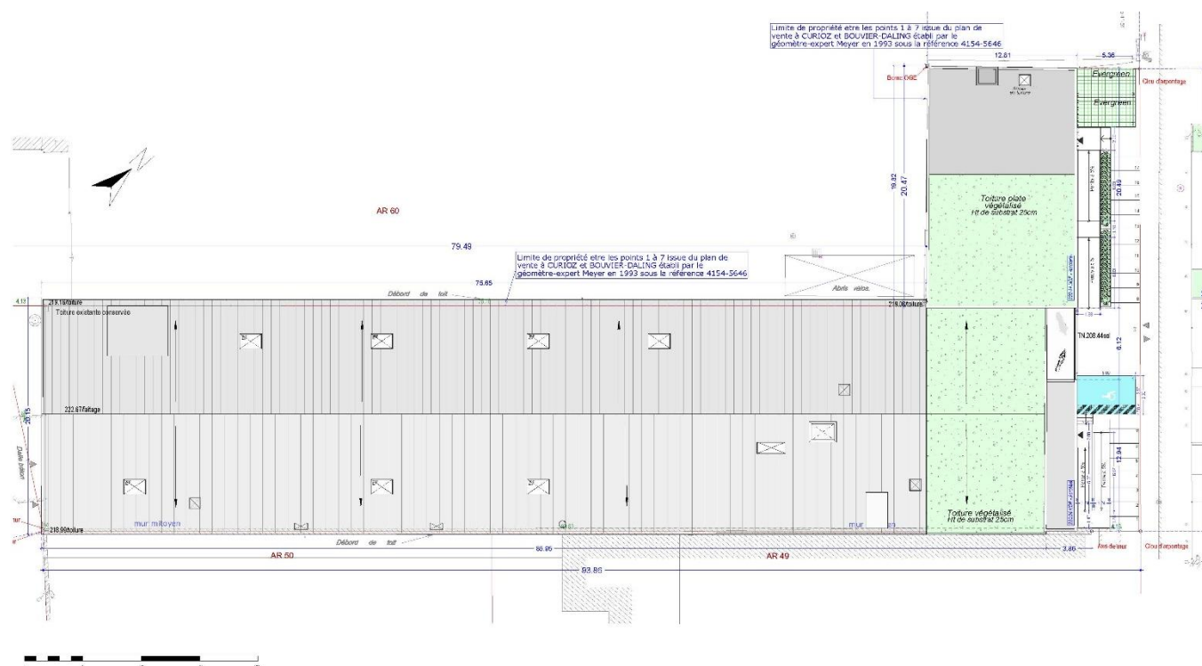
Plan de masse du projet – Source : Arch'Ingenierie
