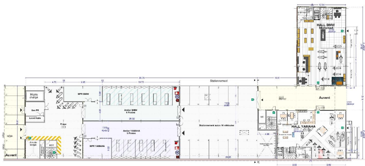
Plan de RDC du projet – Source : Arch'Ingenierie
