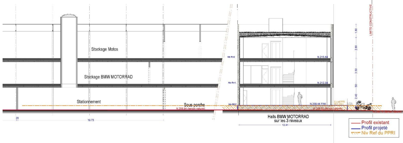
Coupes du projet – Source : Arch'Ingenierie
