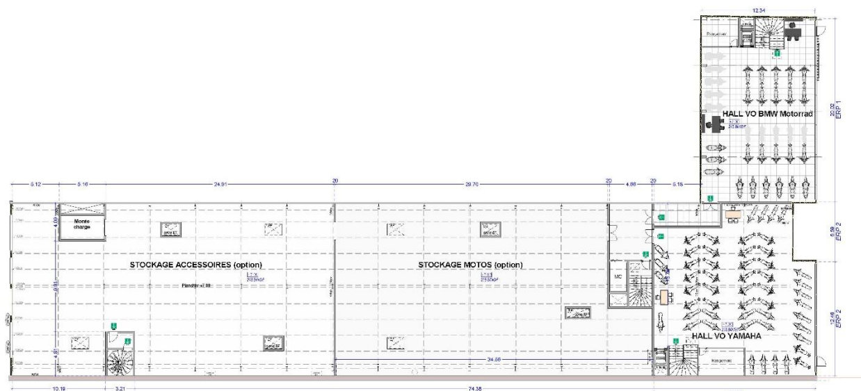
Plan de R+2 du projet – Source : Arch'Ingenierie
