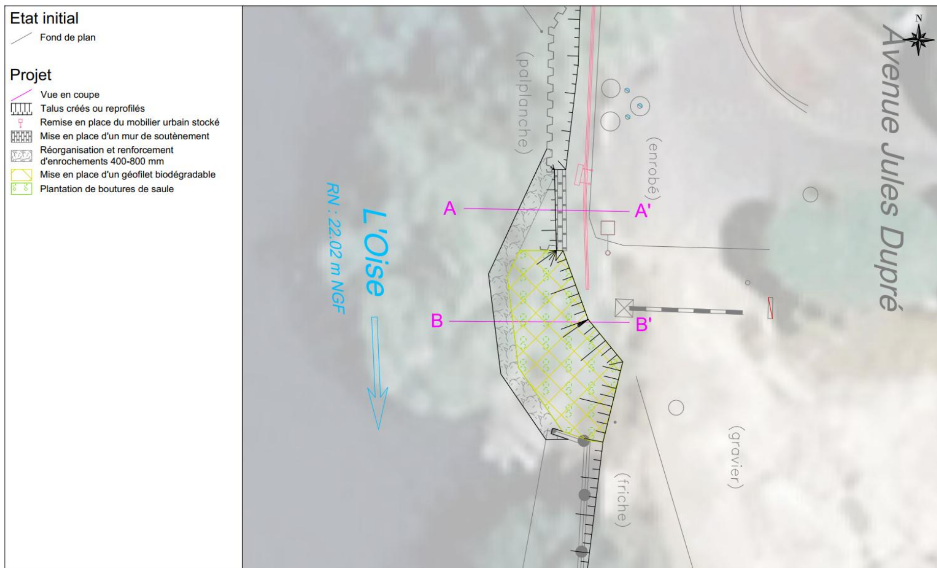
Figure 8 : Plan masse du projet sur le site de L'Isle-Adam.
