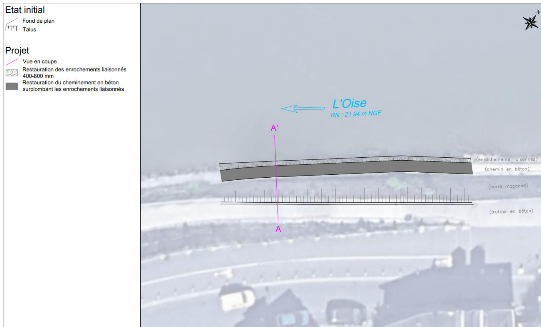
Figure 10 : Plan masse du projet sur le site de Saint-Ouen-l'Aumône.
