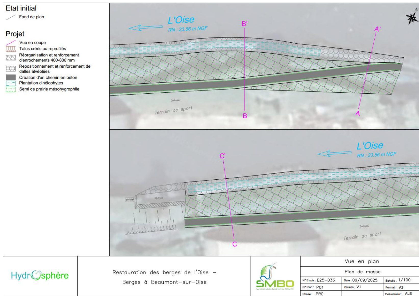
Figure 6 : Plan masse du projet sur le site de Beaumont-sur-Oise.
