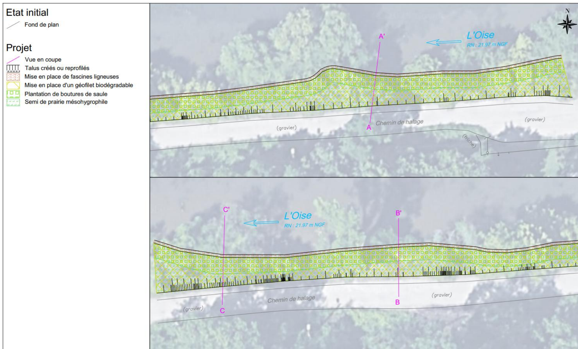
Figure 9 : Plan masse du projet sur le site de Méry-sur-Oise.
