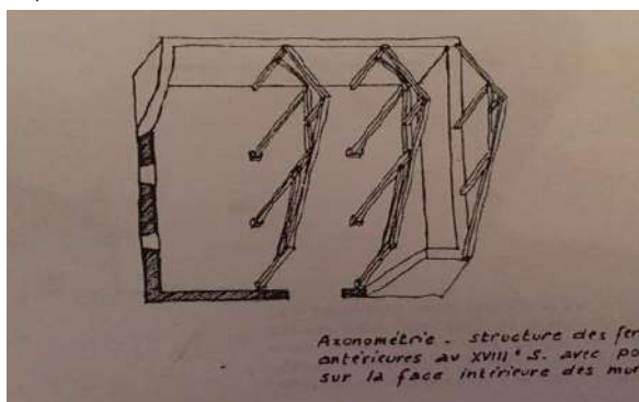
charpente qui repose sur des "hommes debout", en sapin, avec délimitation des 3 travées
