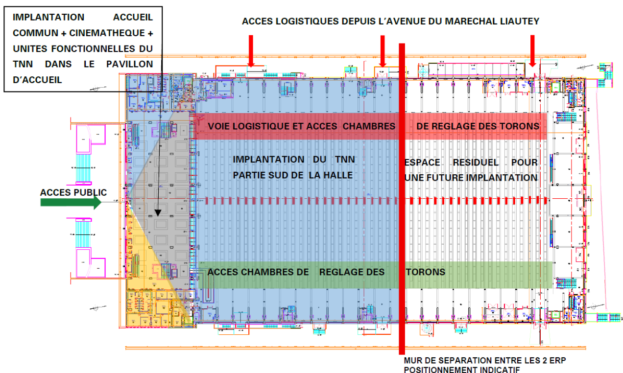
Plan masse et organisation interne du PEX
