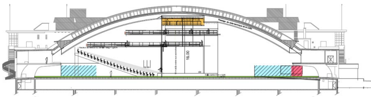
Vue en coupe – Aménagement intérieur du théâtre
