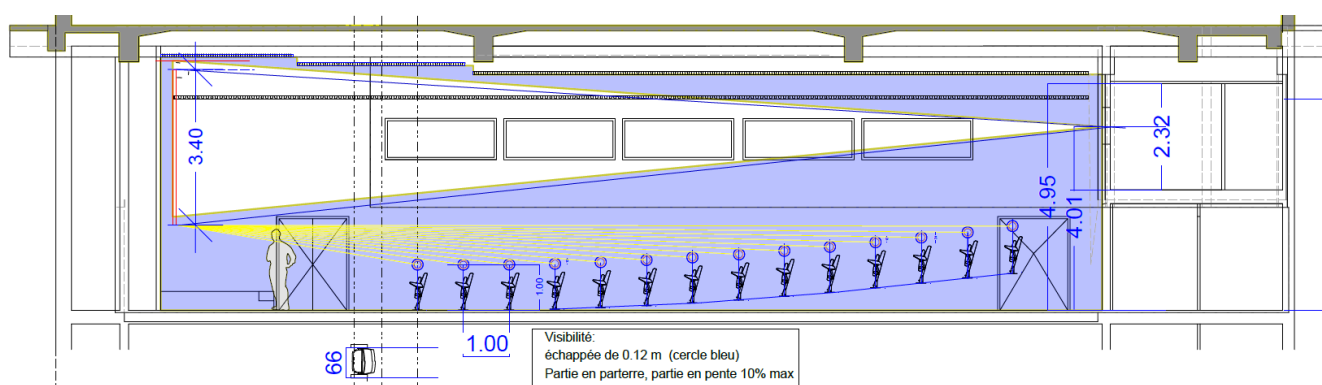
Vue en coupe de la salle de projection
