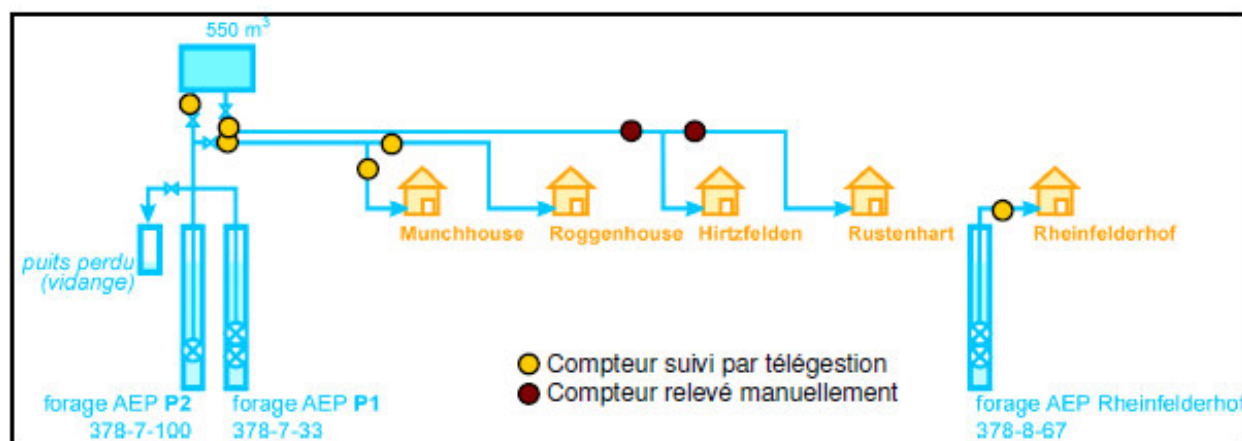
Représentation schématique du réseau d'adduction du SIAEP de Munchhouse et Environs
