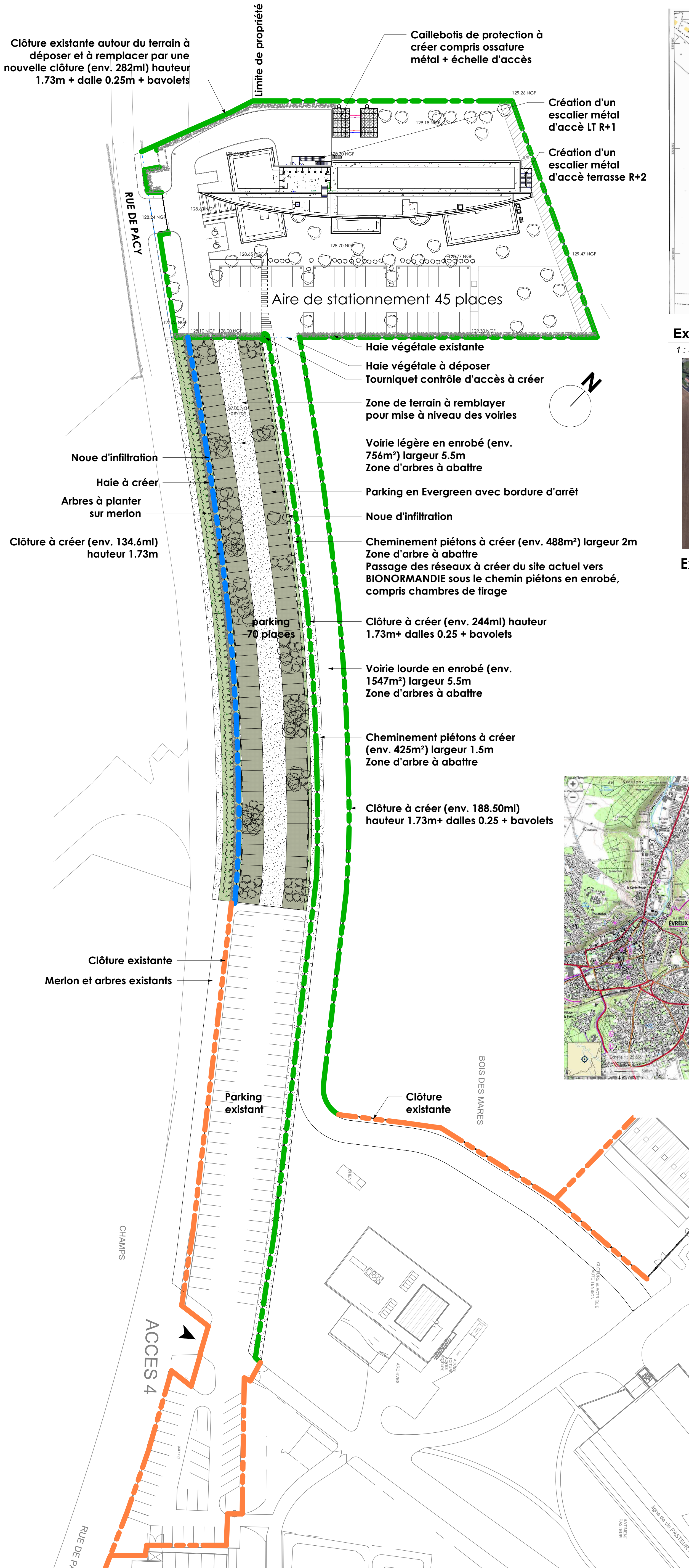
Plan de masse d'ensemble
