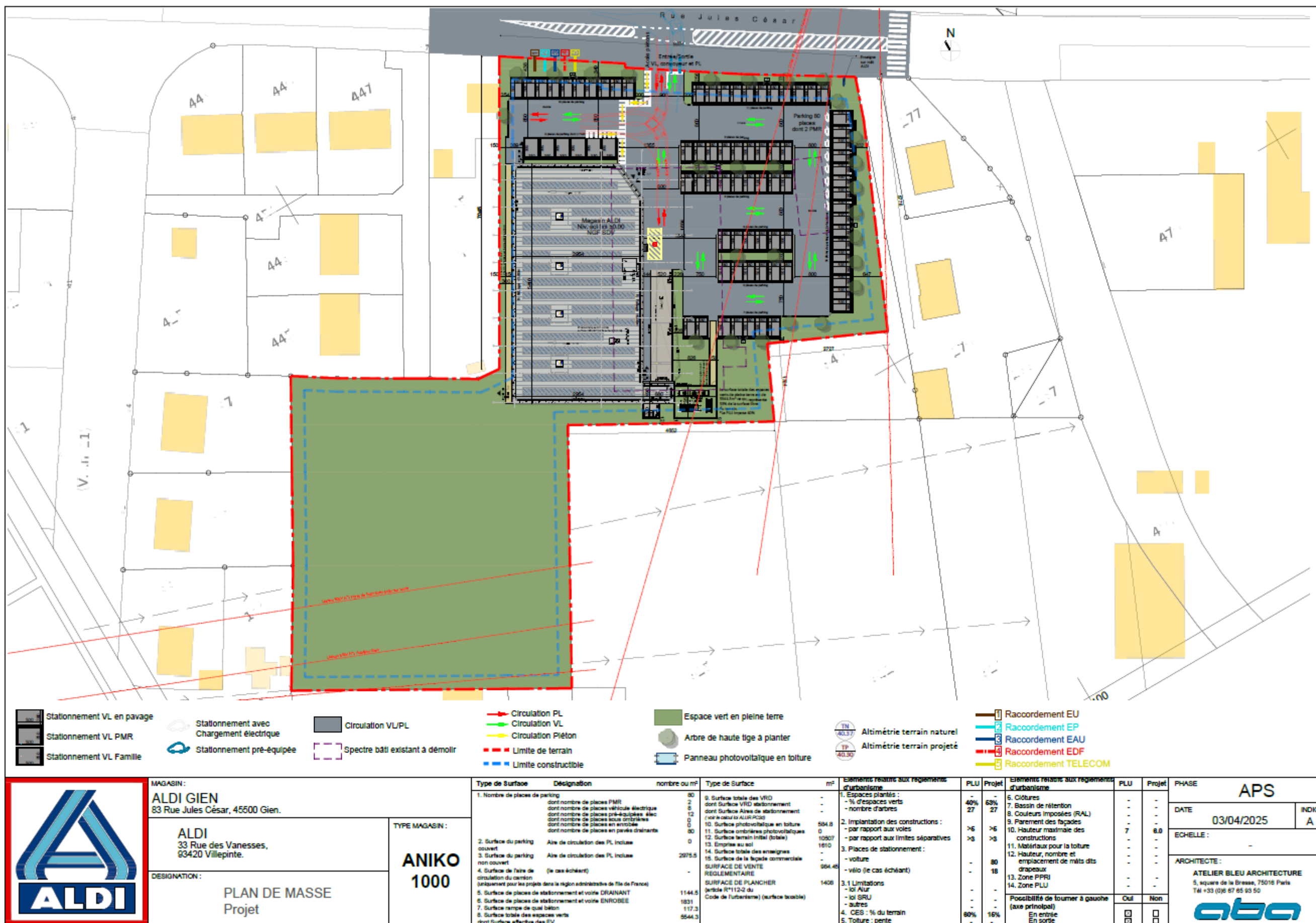
Plan masse du projet Source : Aldi Immobilier
