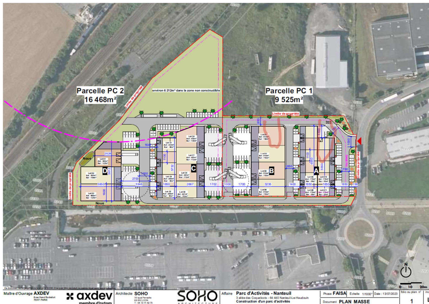
Figure 3 : Plan de masse du projet (source : AXDEV)
