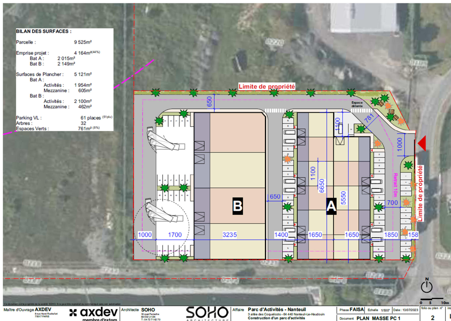
Figure 4 : Plan de masse PC1 (source : AXDEV)
