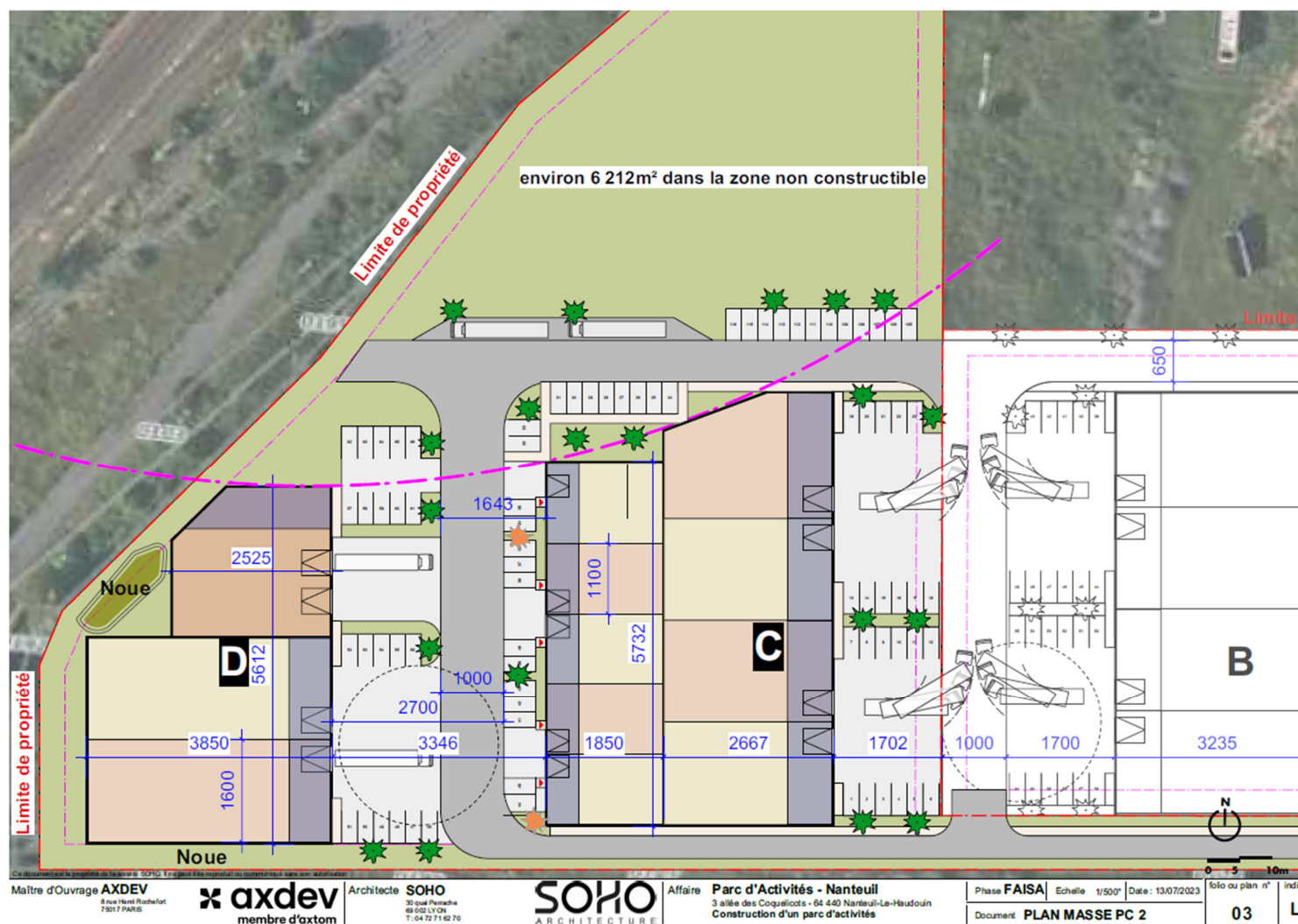
Figure 5 : Plan de masse PC2 (source : AXDEV)
