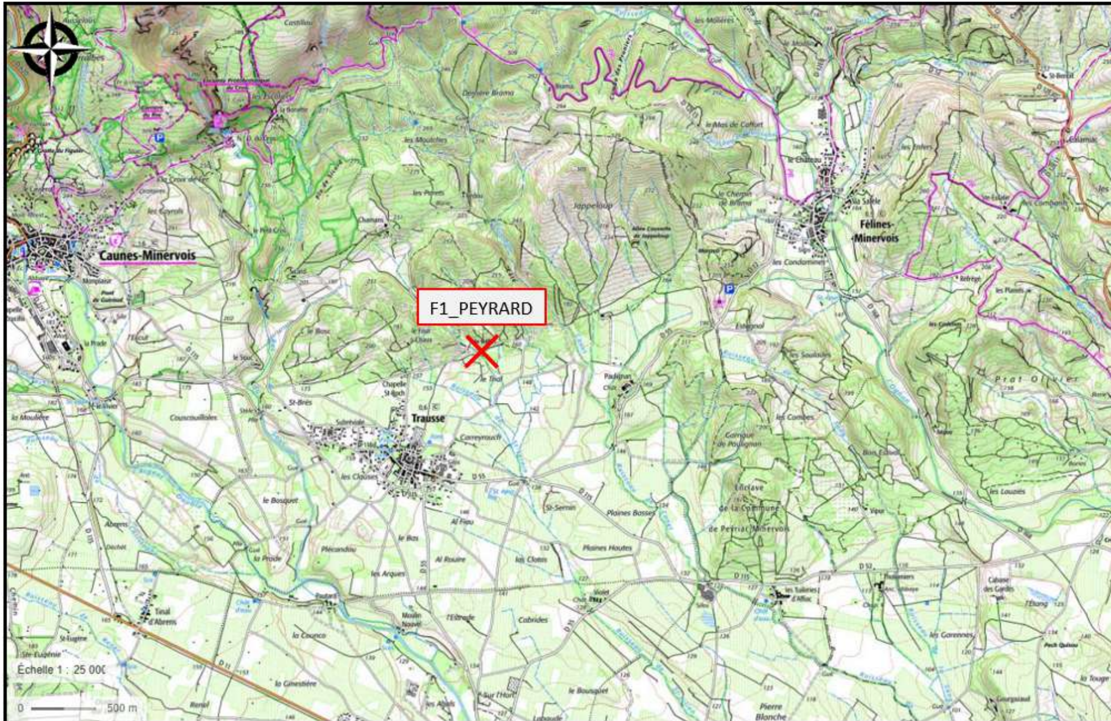
Plan de situation au 1/25 000 du forage F1_Peyrard (source: géoportail )
