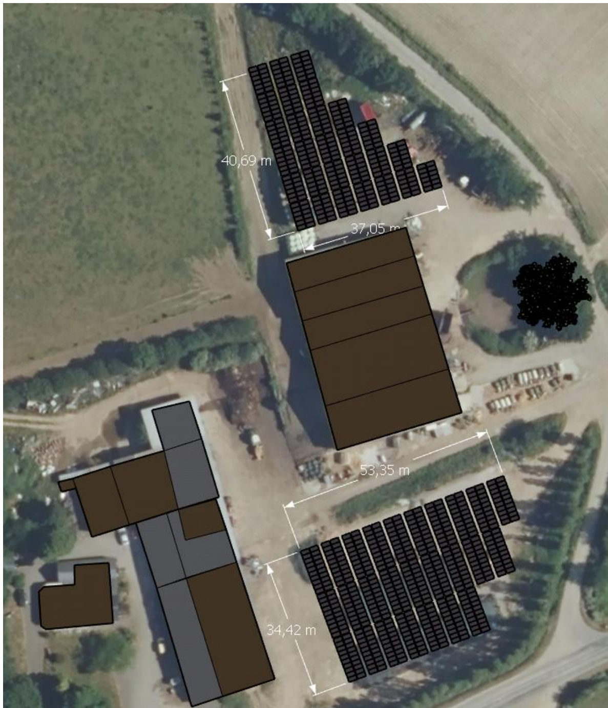
Installation de production d'électricité à partir d'énergie solaire / plan de calpinage – 1 :100- vus satellite
