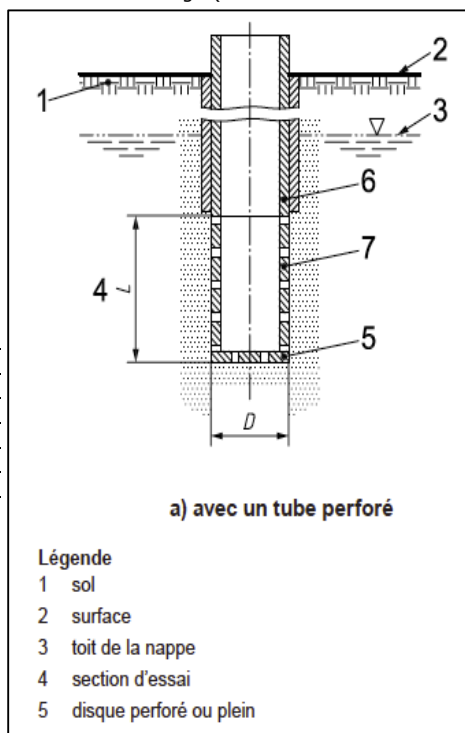
Schéma de l'ouvrage (norme NF EN ISO 22282-2)
