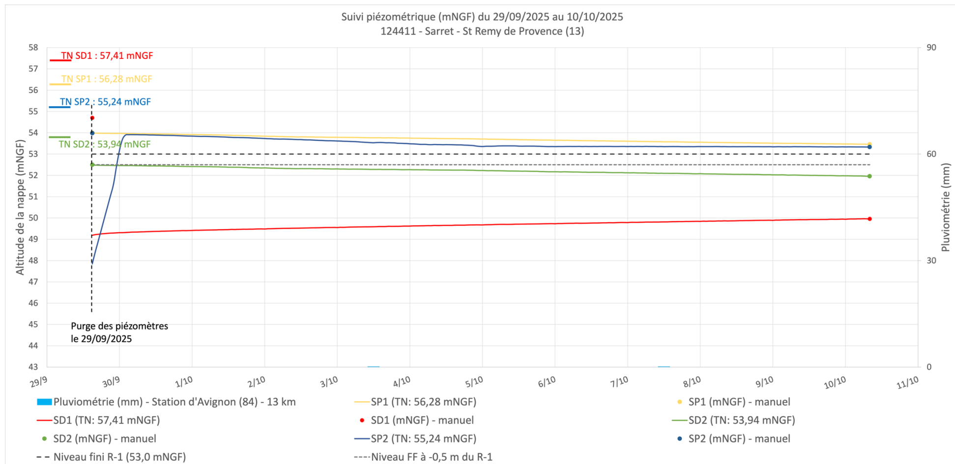
Figure 15 : Suivi piézométrique au droit du site
