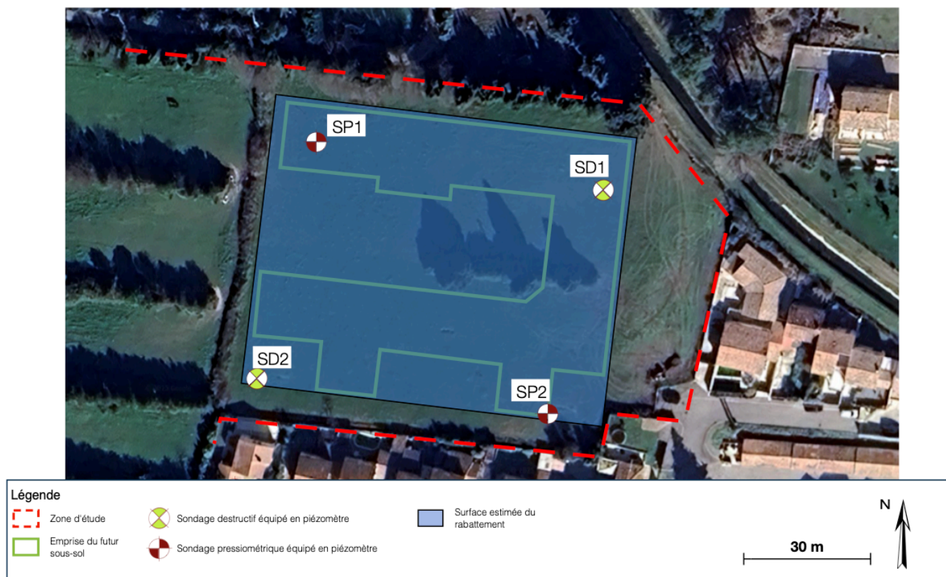
Figure 18 : Surface théorique estimée concernée par un rabattement
