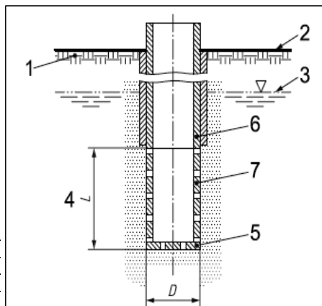
a) avec un tube perforé
