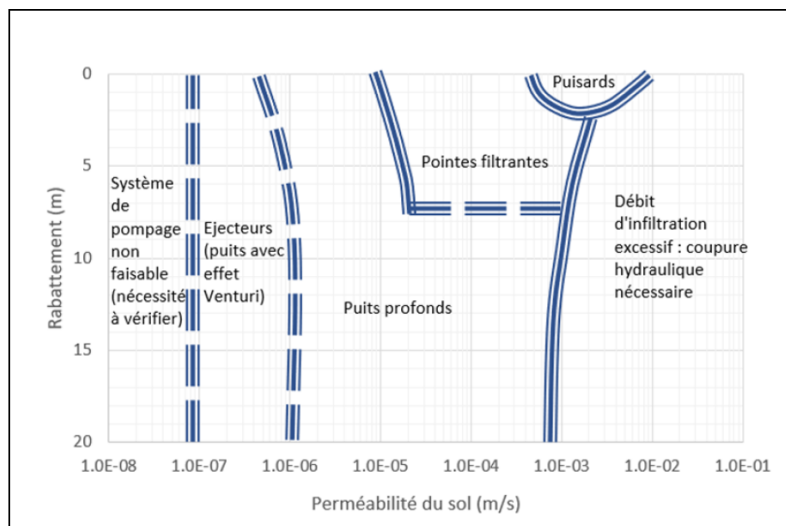
Figure 19 : Système de pompage selon le document du CIRIA C515 (2000), modifié par l'auteur (Pré-dimensionnement d'un système de pompage - Grégory Meyer)
