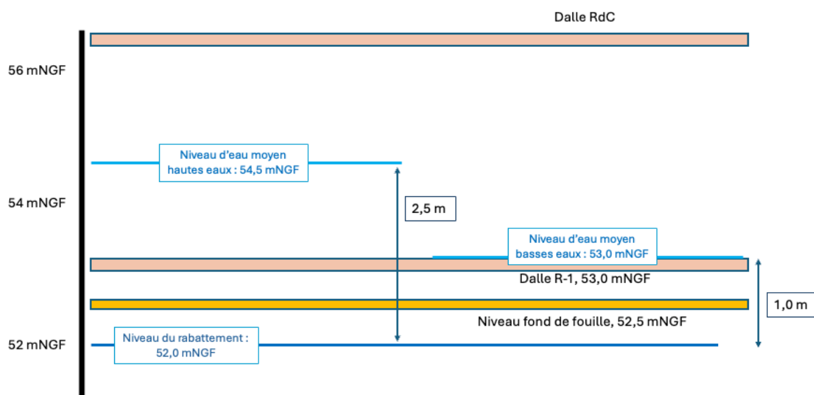
Figure 17 : Synthèse de l'interaction de la nappe avec le projet en phase chantier
