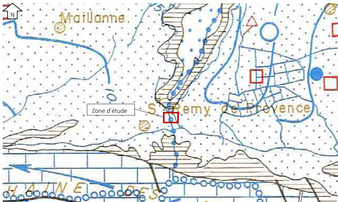
Figure 11 : Carte hydrogéologique des Bouches du Rhône de 1972 (BRGM)
