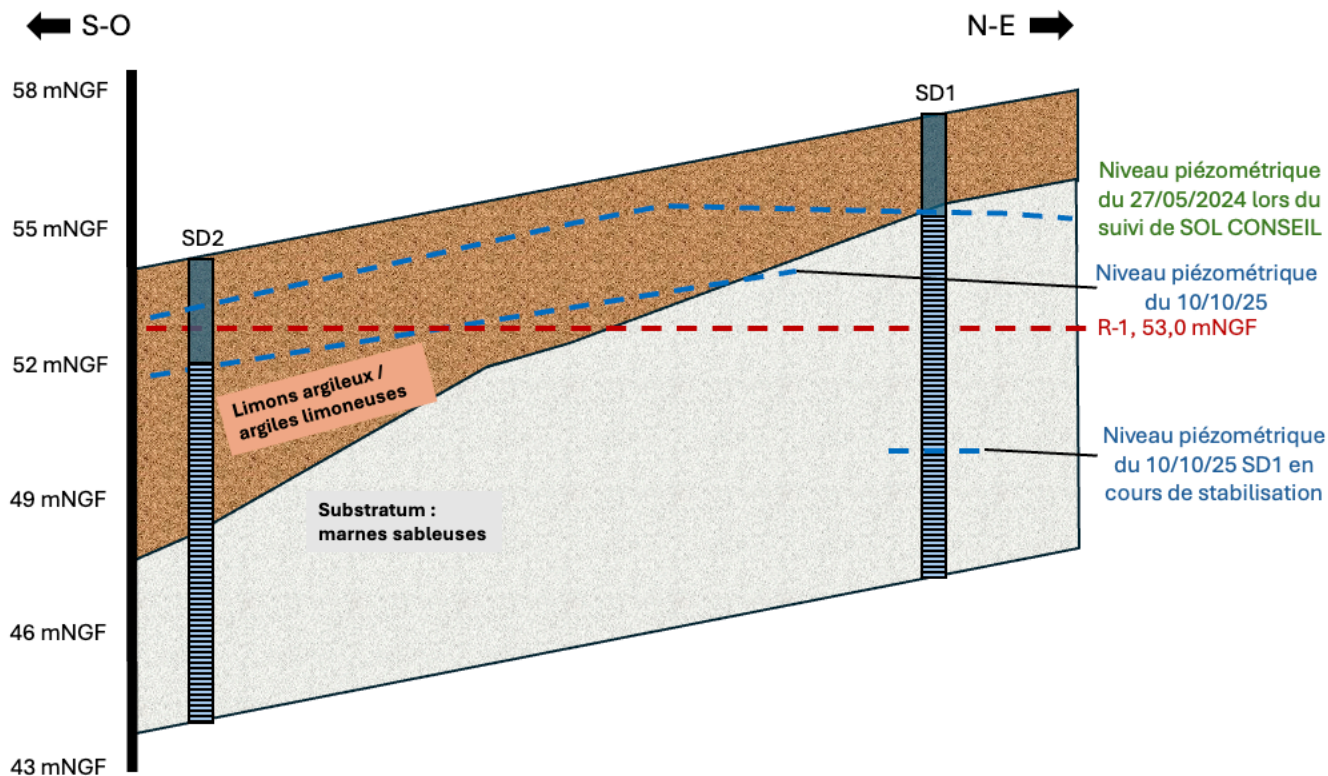
Figure 16 : Synthèse hydrogéologique au droit du site
