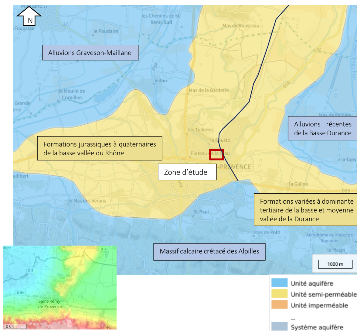
Figure 9 : Extrait de la carte BDLISA autour de la zone d'étude et topographie de la zone (topographic-map.com)
