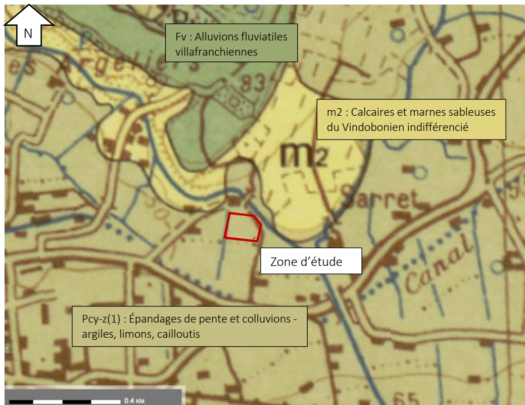
Figure 4 : Carte géologique au 1/50 000ème aux alentours du site
