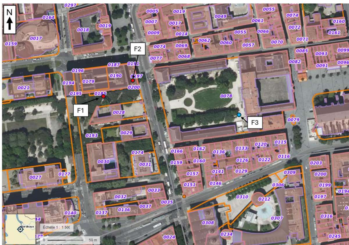
Figure 2: Localisation des puits géothermiques sur photographie aérienne avec cadastre (source : Géoportail)
