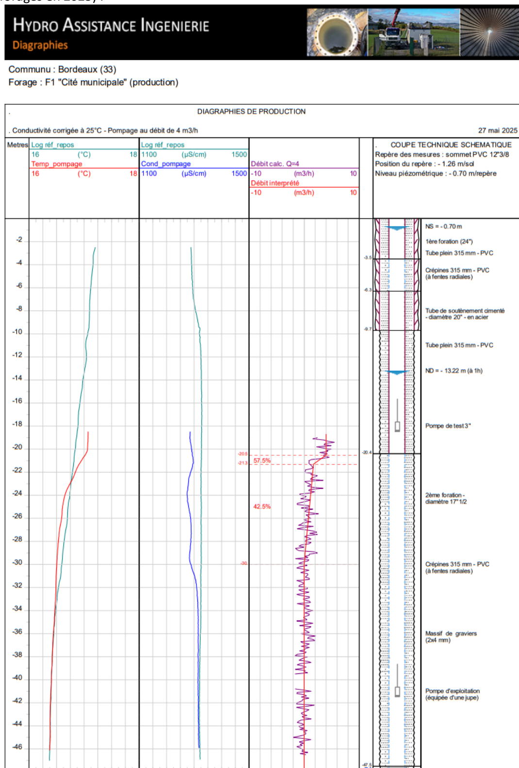
Figure 3 : Coupe technique et synthétique des diagraphies du forage F1 (mai 2025 – rapport Hydro-Assistance)
