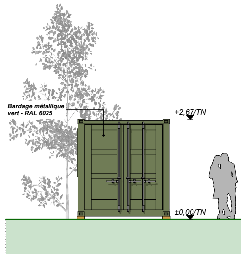
Façade NORD - OUEST
