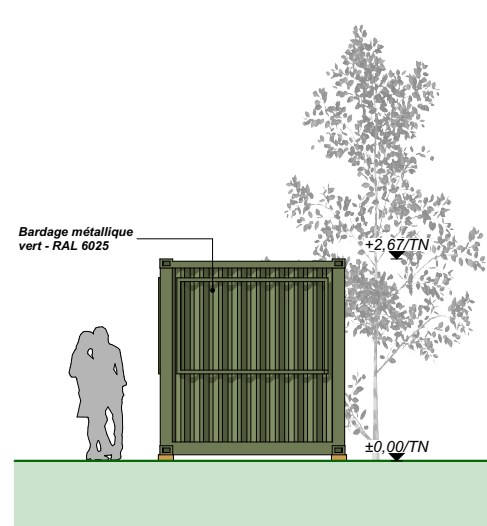
Façade OUEST
