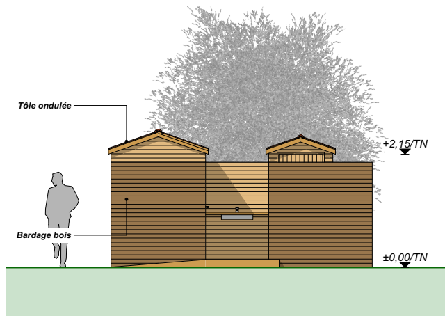
Façade SUD - OUEST
