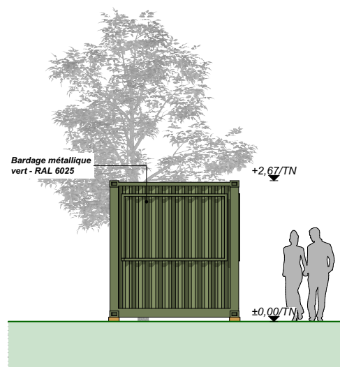
Façade SUD - EST
