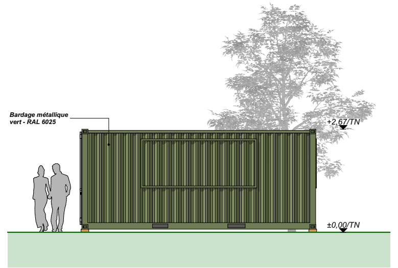
Façade NORD
