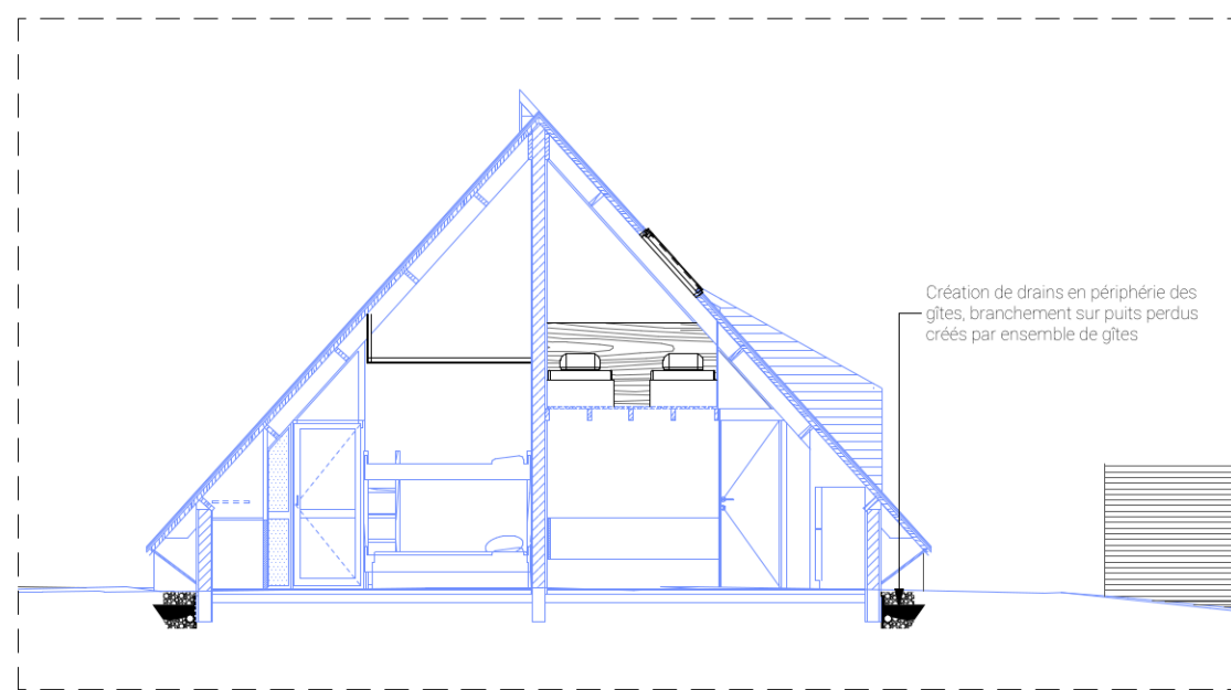
Coupe AA
