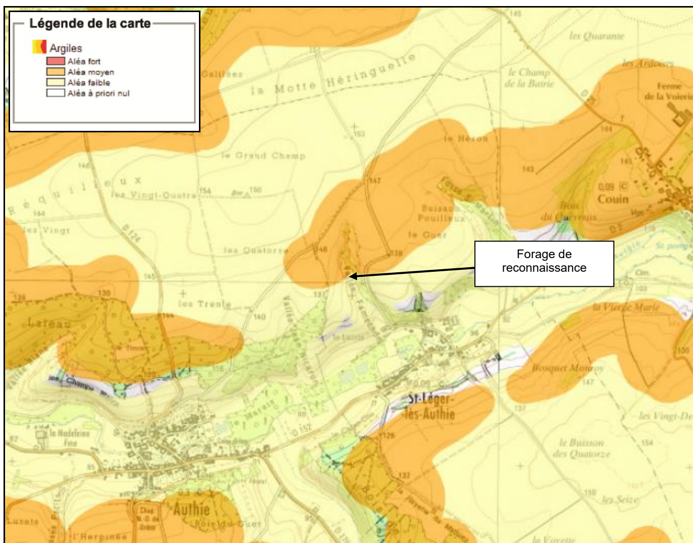
Figure 10 : Carte de l'aléa retrait-gonflement des sols argileux (1/25000 ème ) Source BRGM
