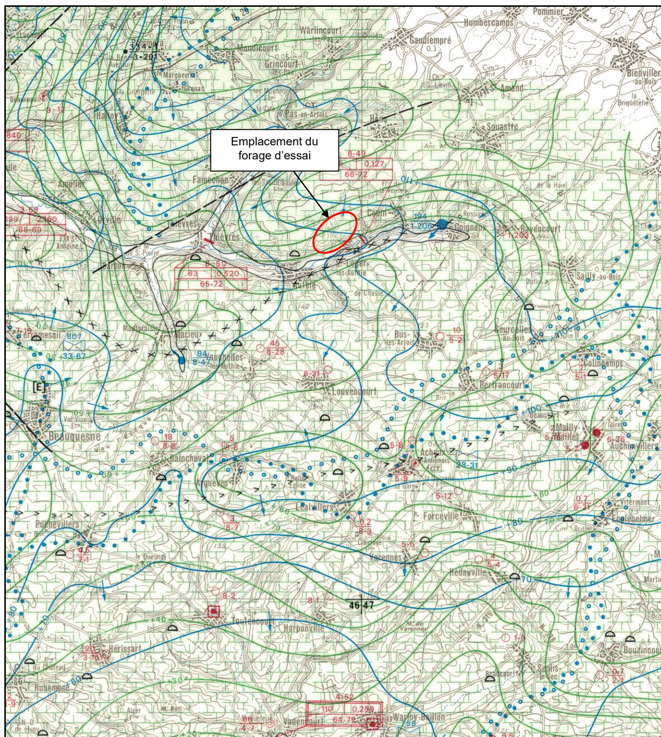
Figure 8 : Extrait de la carte hydrogéologique de la Somme (1/100 000 ème )
