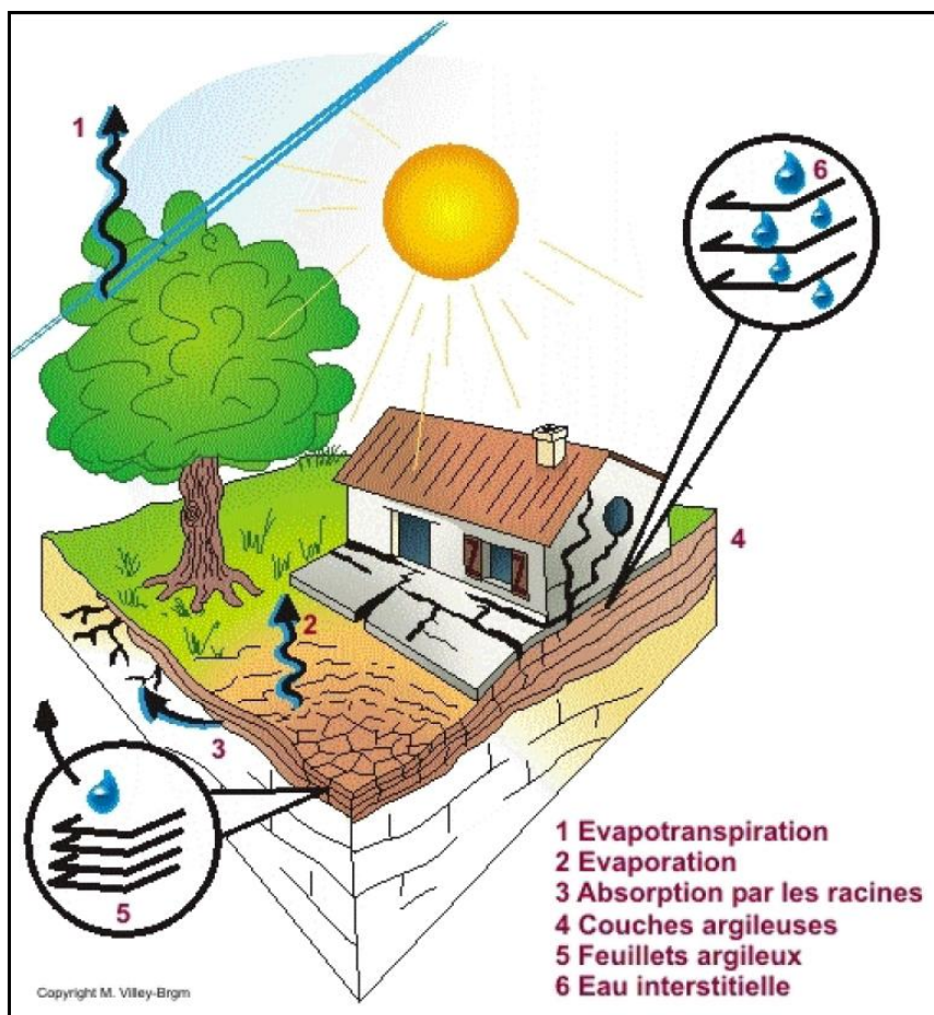
Figure 9 : Dessiccation des sols argileux en période sèche
