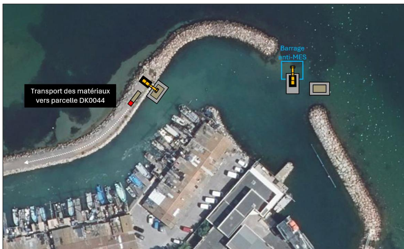
Figure 3 : Schéma de principe des travaux de dragage mécanique
