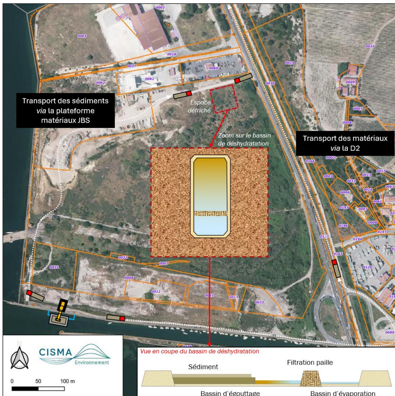
Figure 4 : Schéma de principe des opérations de déshydratation des matériaux sur la parcelle DK0044
