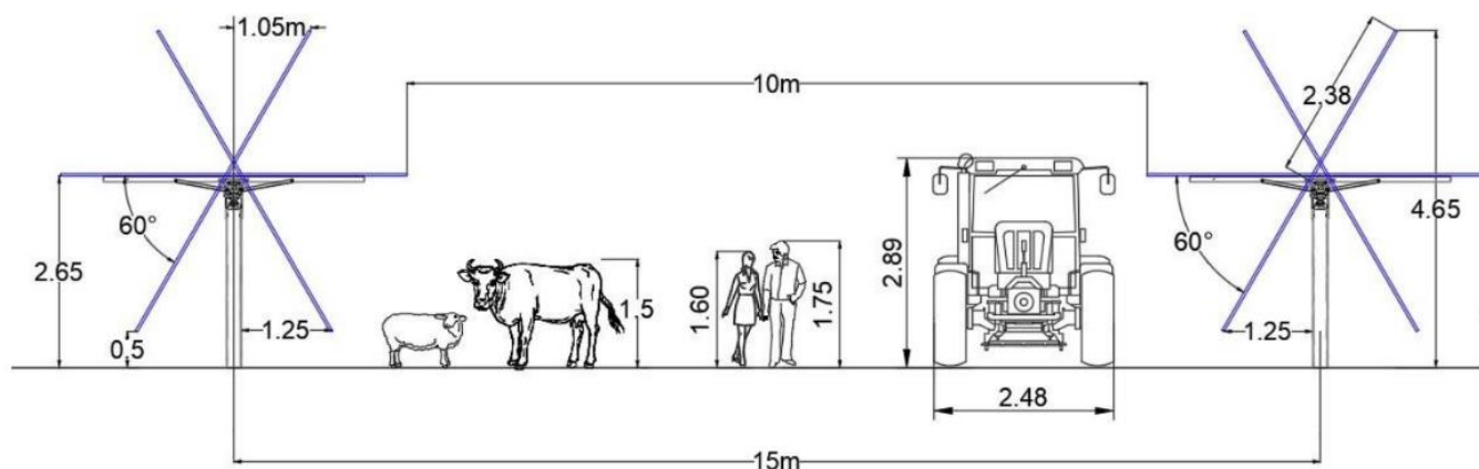
Figure 1 : Schéma de principe d'une ombrière (source : TSE)
