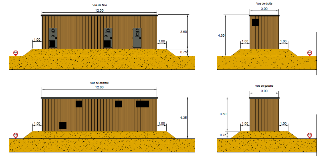
Figure 2 : façades du poste de livraison (source : TSE)
