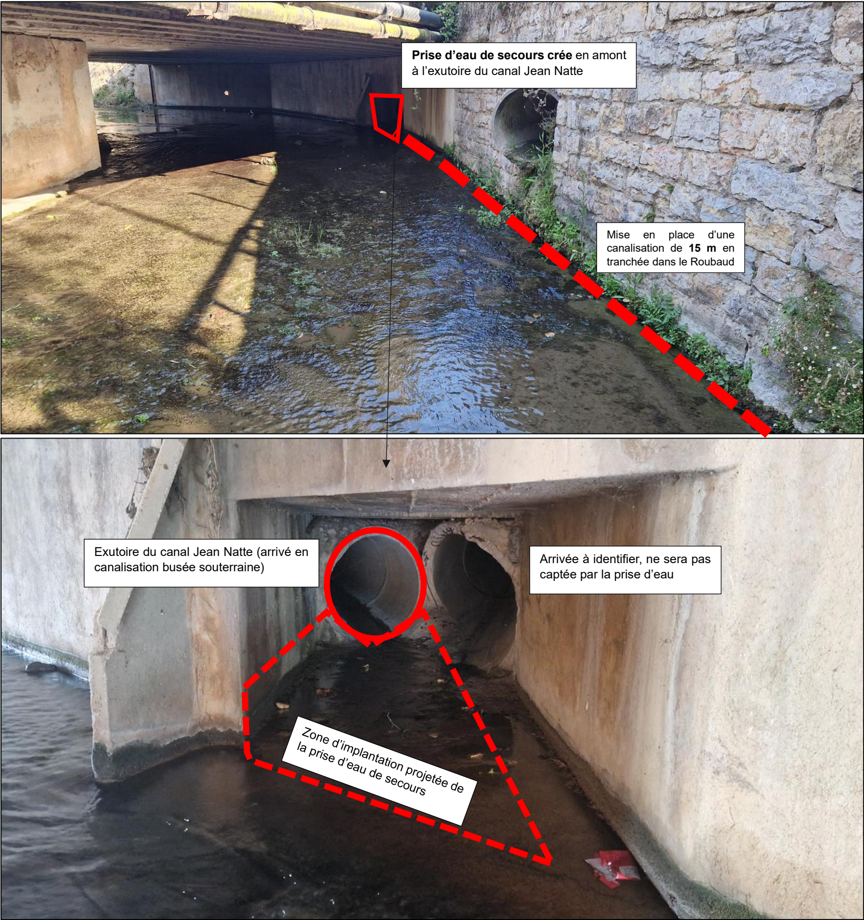
Figure 2 : Annexe 4 - photographies datées de la zone de travaux au niveau de la prise d'eau de secours
