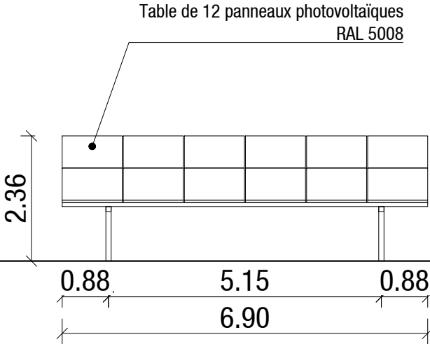
FAÇADE SUD
