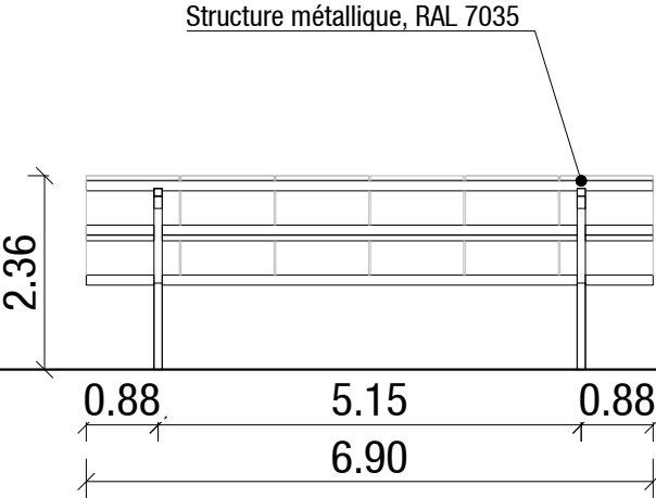
FAÇADE NORD
