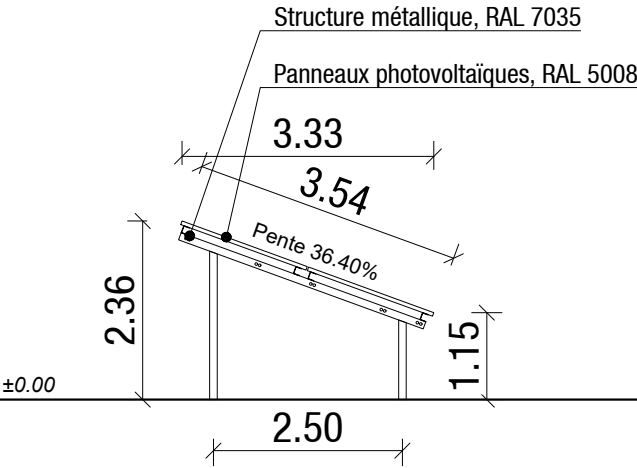
FAÇADE OUEST
