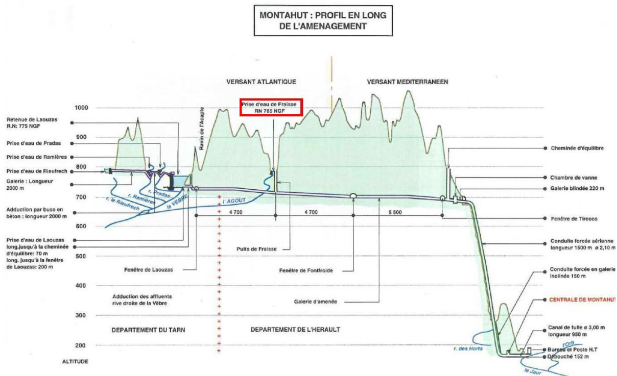
Figure 3 Vue schématique des principaux aménagements de Montahut
