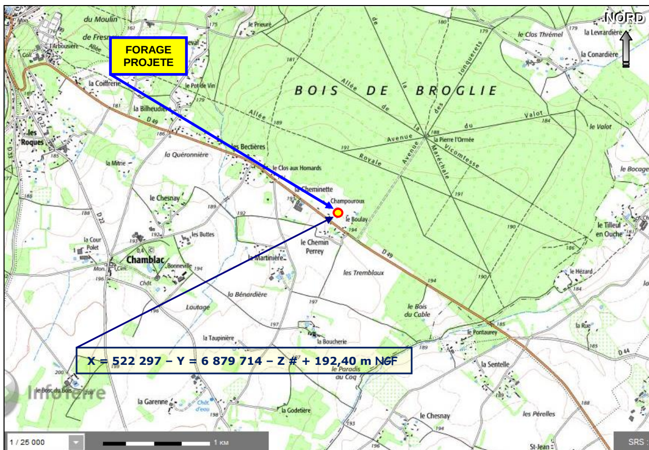
Situation du forage projeté par M r François ENCHERY au lieu-dit du BOULEY à CHAMBLAC (27) sur un extrait de carte topographique de l'IGN à 1/25 000° (Extrait de : infoterre.brgm.fr)
