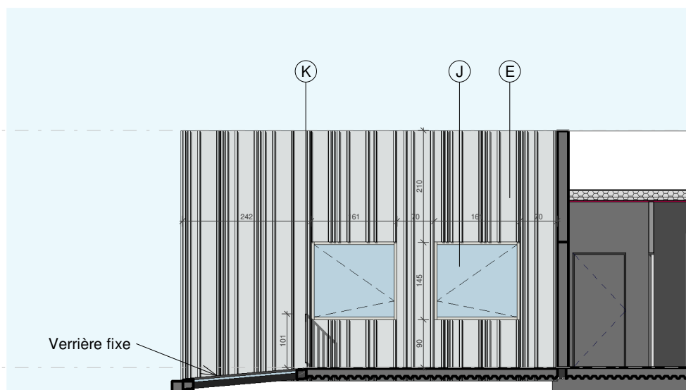
4 PATIO FACADE 4 1 : 100
