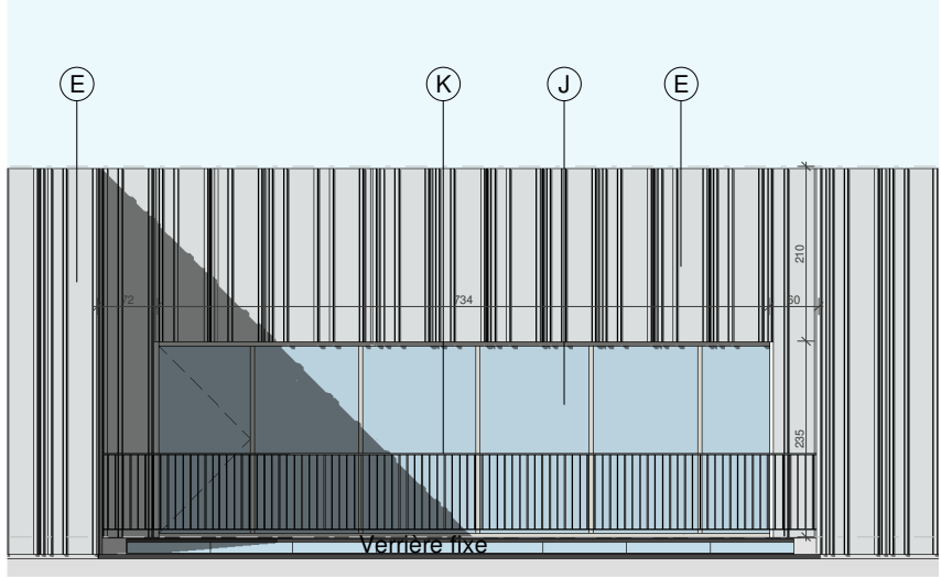
2 PATIO FACADE 2 1 : 100
