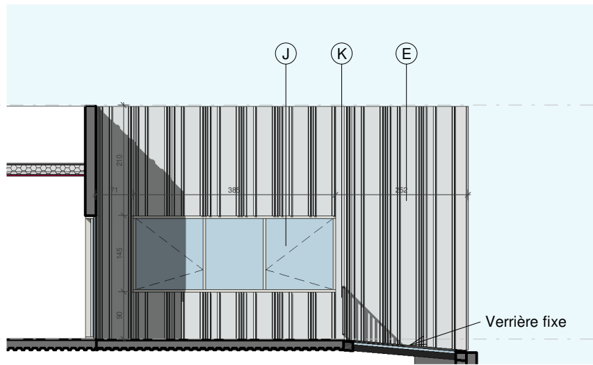
3 PATIO FACADE 3 1 : 100
