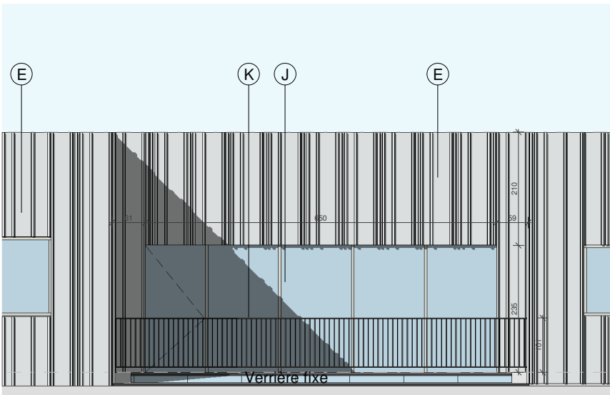
5 PATIO FACADE 5 1 : 100
