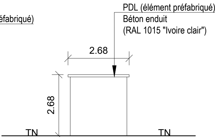
FAÇADE EST
