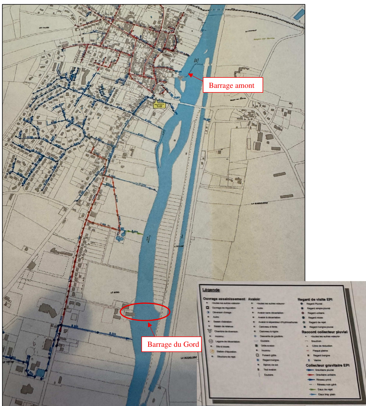
Photo 1 : Plan des réseaux d'eaux pluviales ; 2021 (Source : Mairie)
