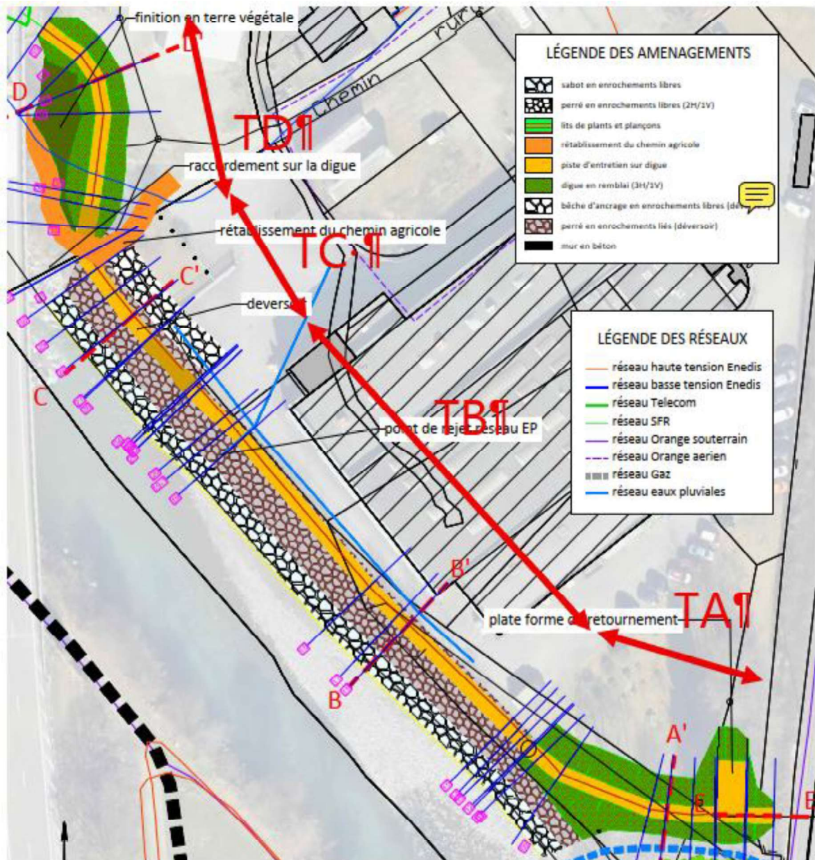
Figure 5 : Plan sur la décomposition du secteur d'étude en quatre tronçons homogènes
