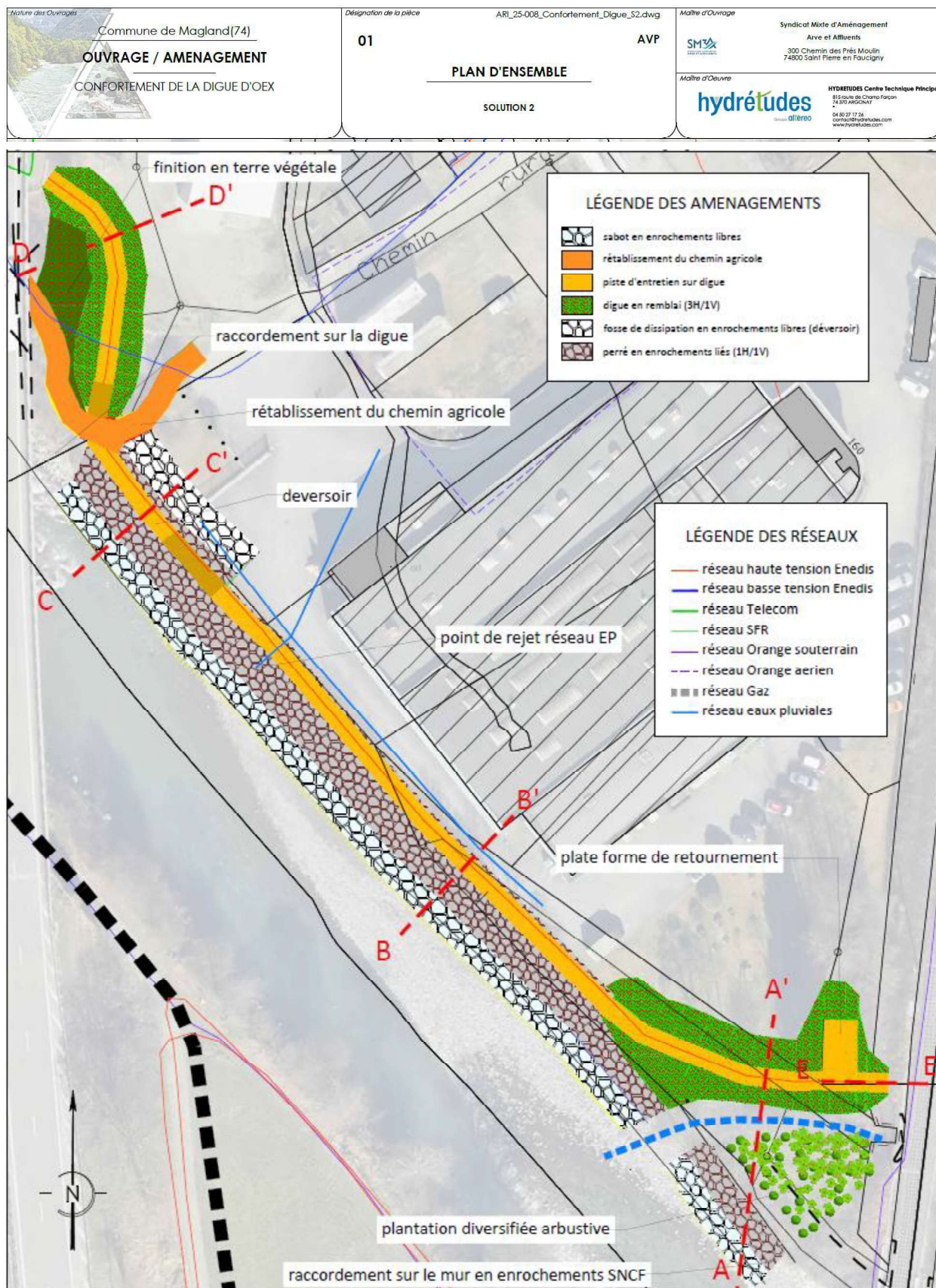
Figure 6 : Solution n°2 – Vue en plan de la digue et du perré en enrochements liés
