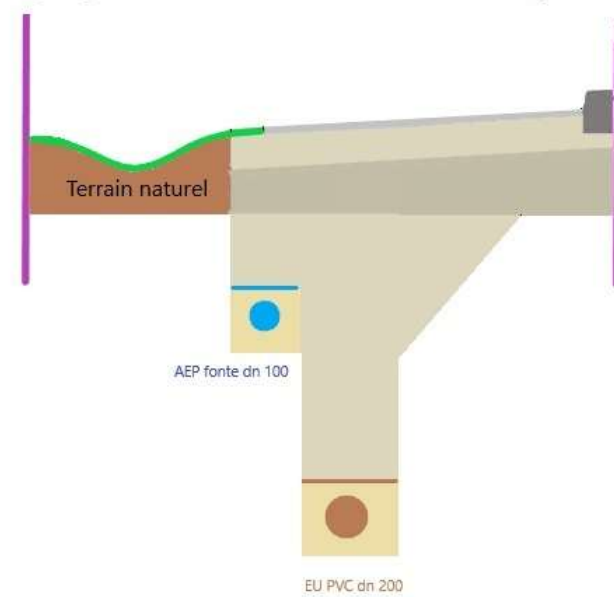
PRINCIPE DE TRANCHEE
