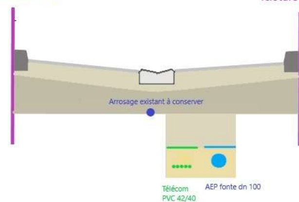
PRINCIPE DE TRANCHEE
