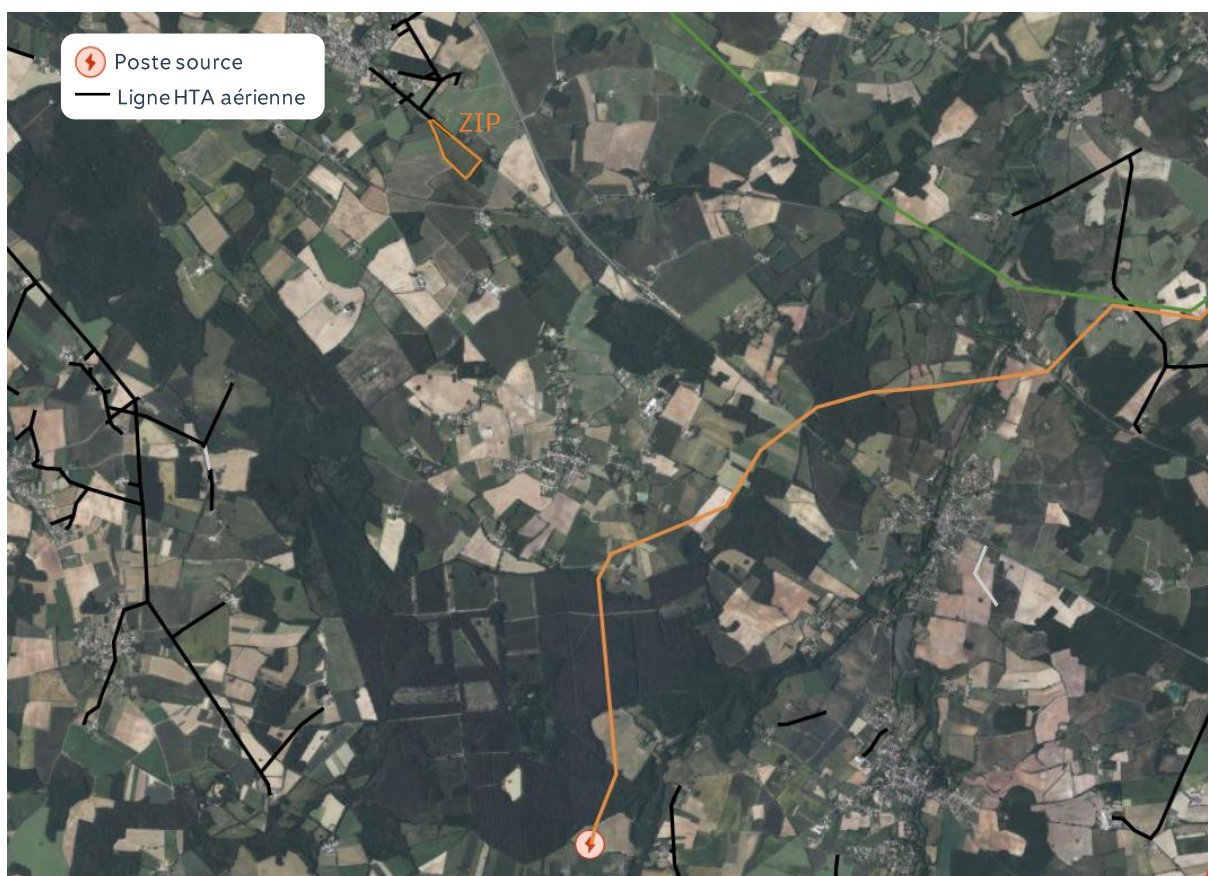
Réseau électrique
