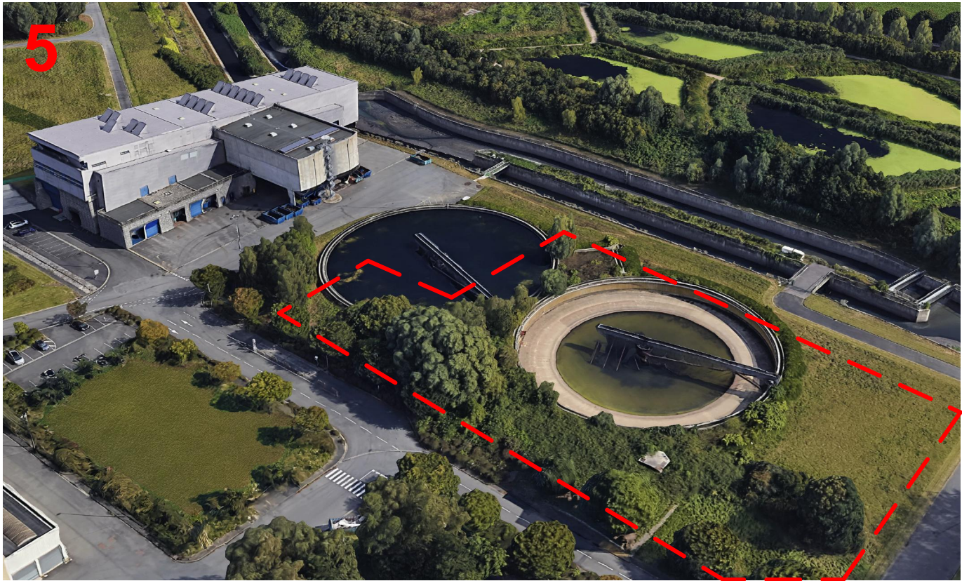
DECANTEURS PRIMAIRES ET CANAL D'ARRIVÉE À DEMOLIR (DEPUIS LE NORD)
