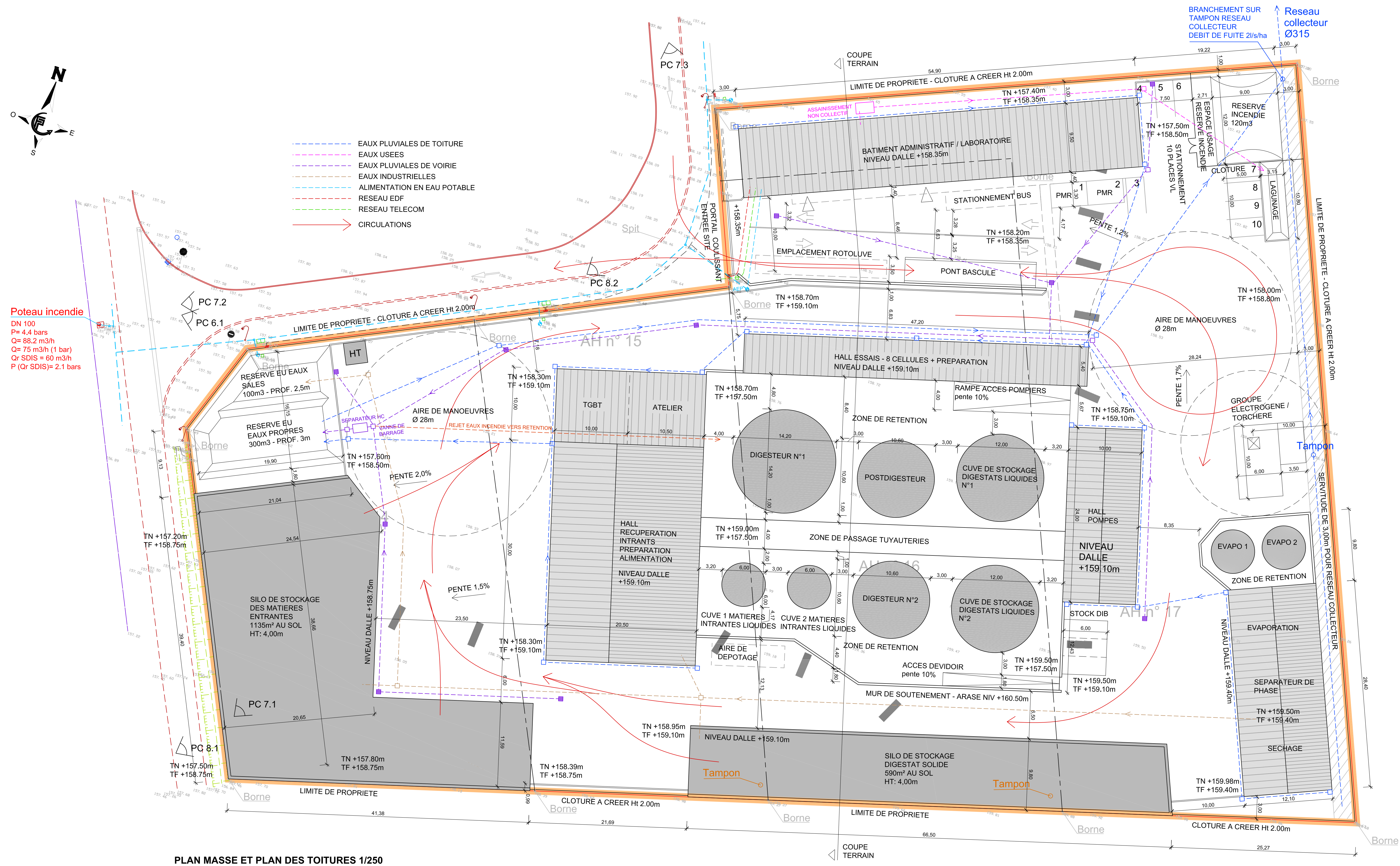
PLAN MASSE ET PLAN DES TOITURES 1/250
