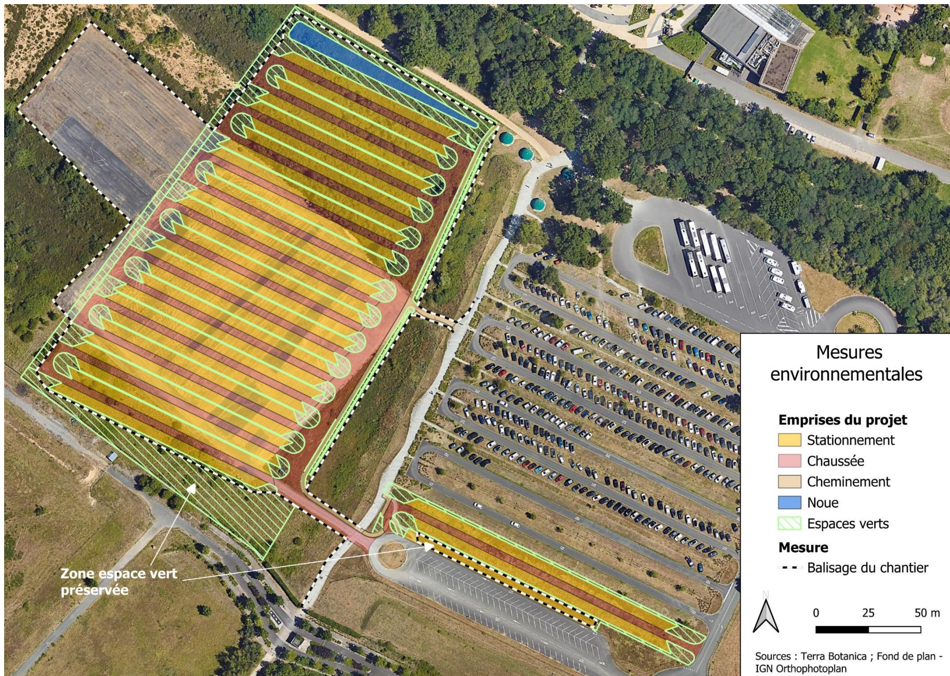
Figure 14 : Localisations des mesures environnementales (zone évitée et balisage chantier)
