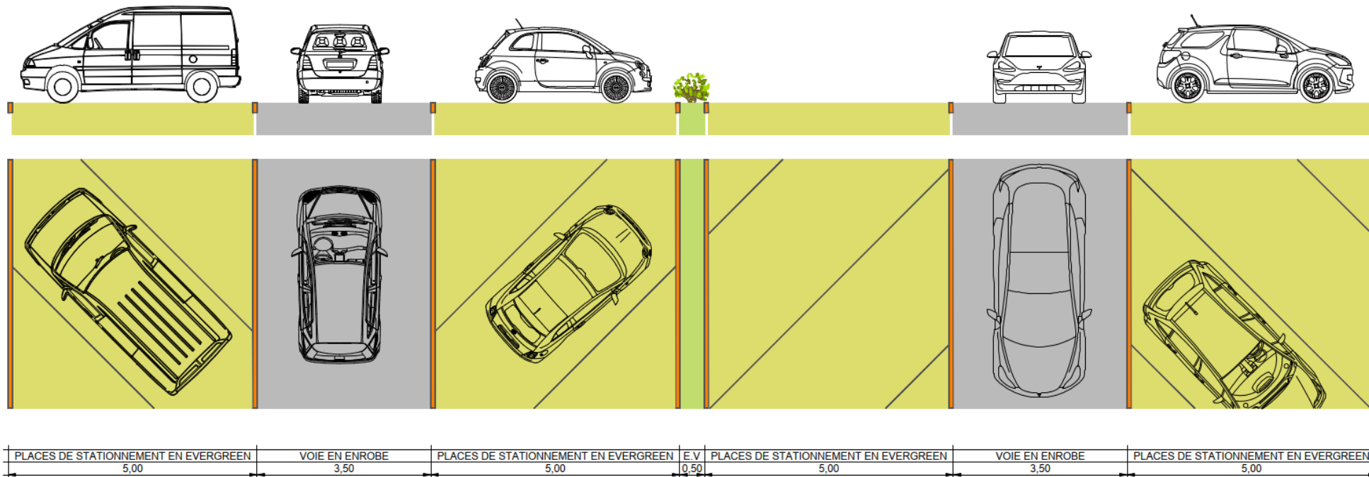
Figure 3 : Coupe de principe du stationnement sur le parking
