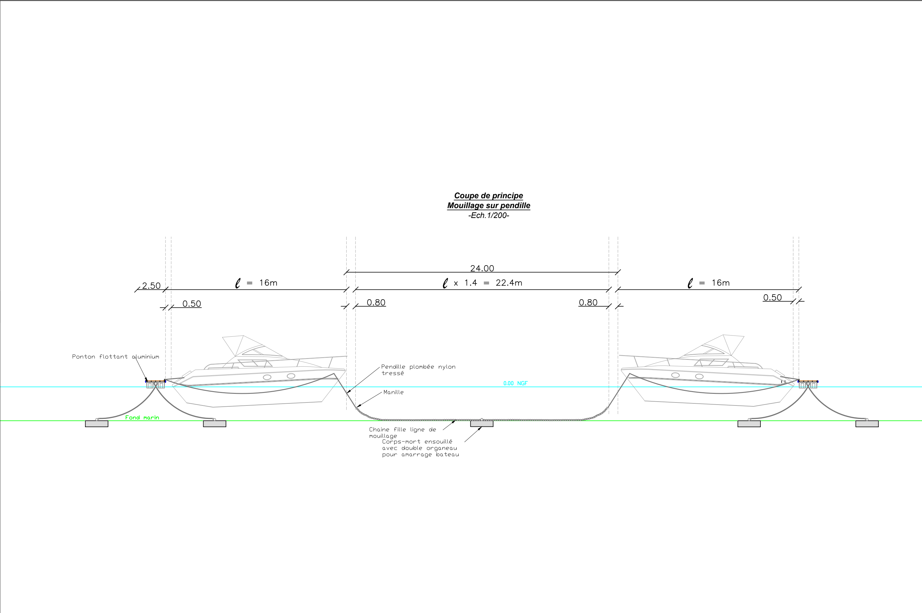
Coupe de principe d'amarrage des bateaux
