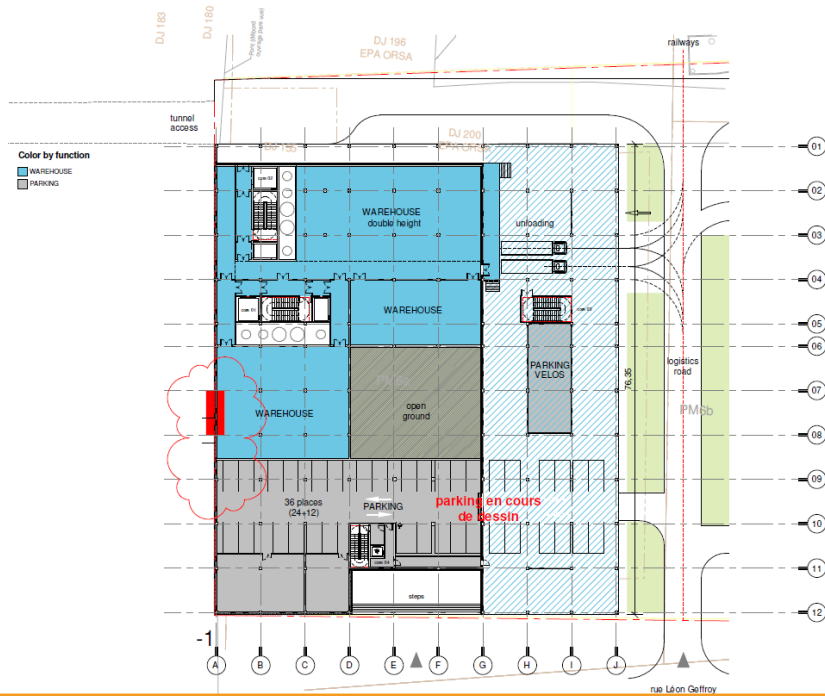
Plan du projet, étage RDC bas (source Richez Associés, 2026)
