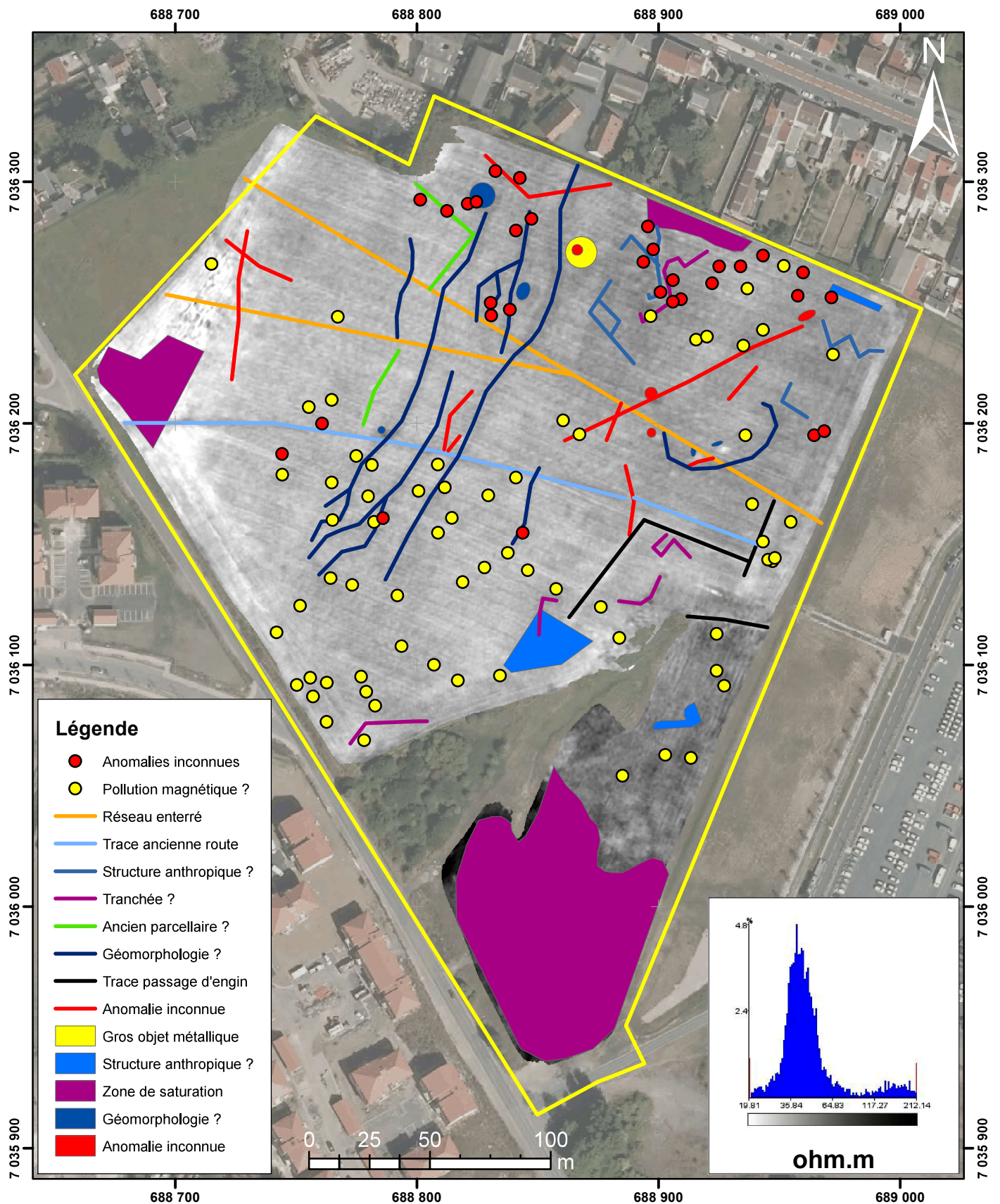
Annexe 12 : Carte d'interprétation supposées des anomalies géophysiques Fond : carte de résistivité ARP 0-100 cm – Echelle : 19.81-212.14 ohm.m
