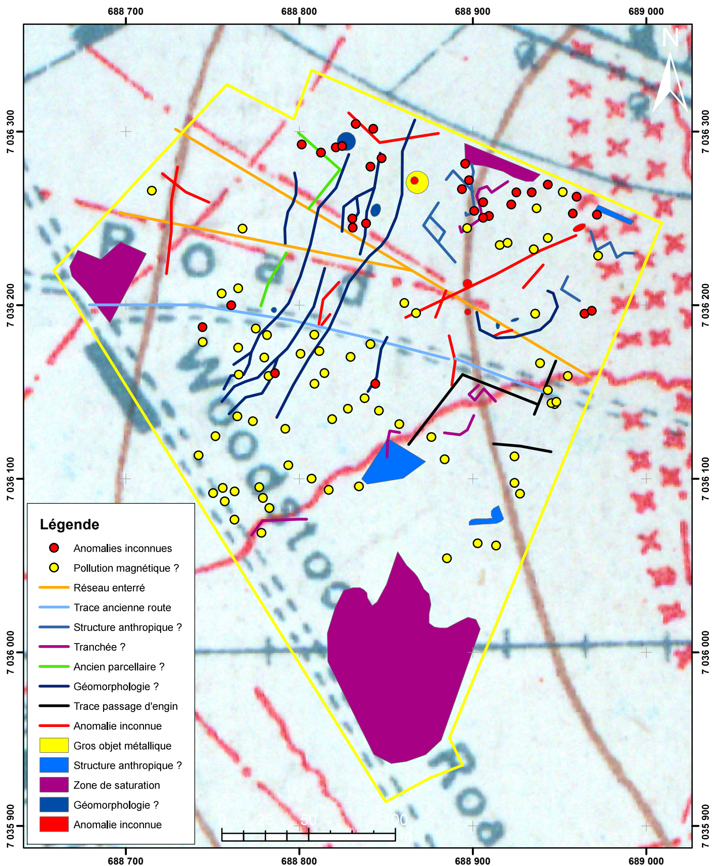
Annexe 13 : Carte d'interprétation supposées des anomalies géophysiques Fond : carte des tranchées en juillet 1917
