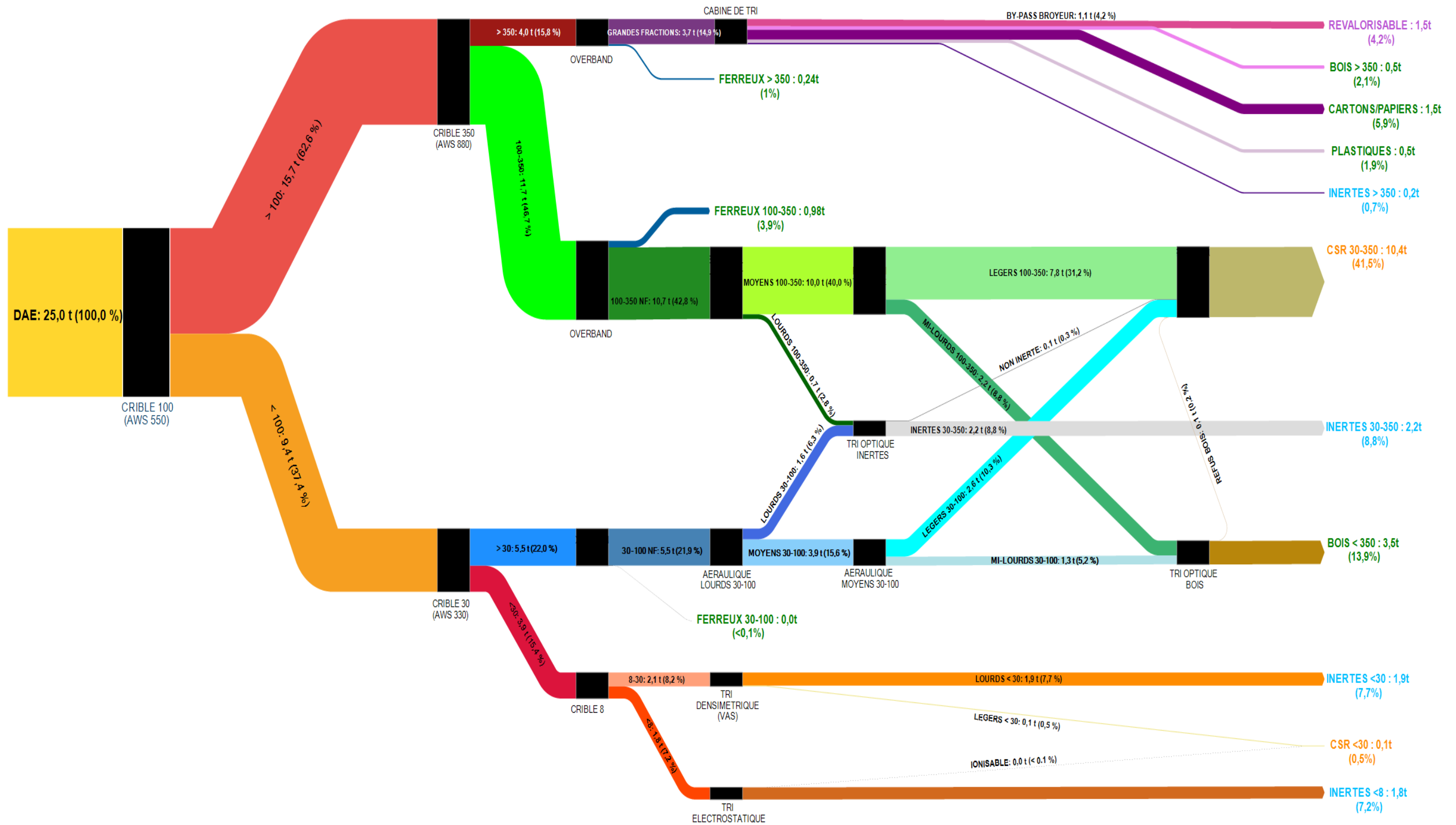
Figure 15 : Diagramme de Sankey – Fractions de sorties
