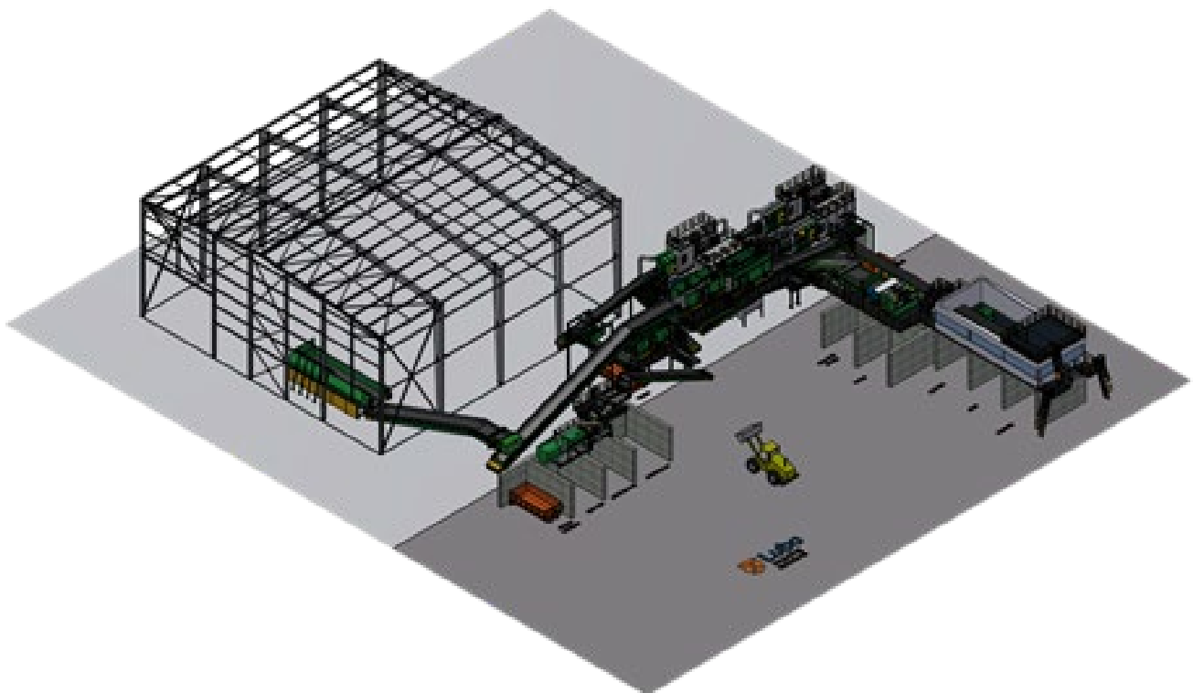
Figure 12 : Aperçu 3D de la chaîne de tri complète
