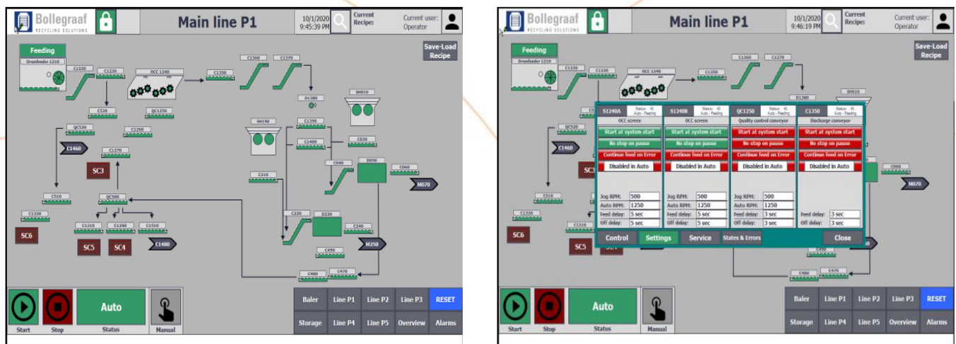
Figure 14 Interface du pupitre de commande de l'installation
