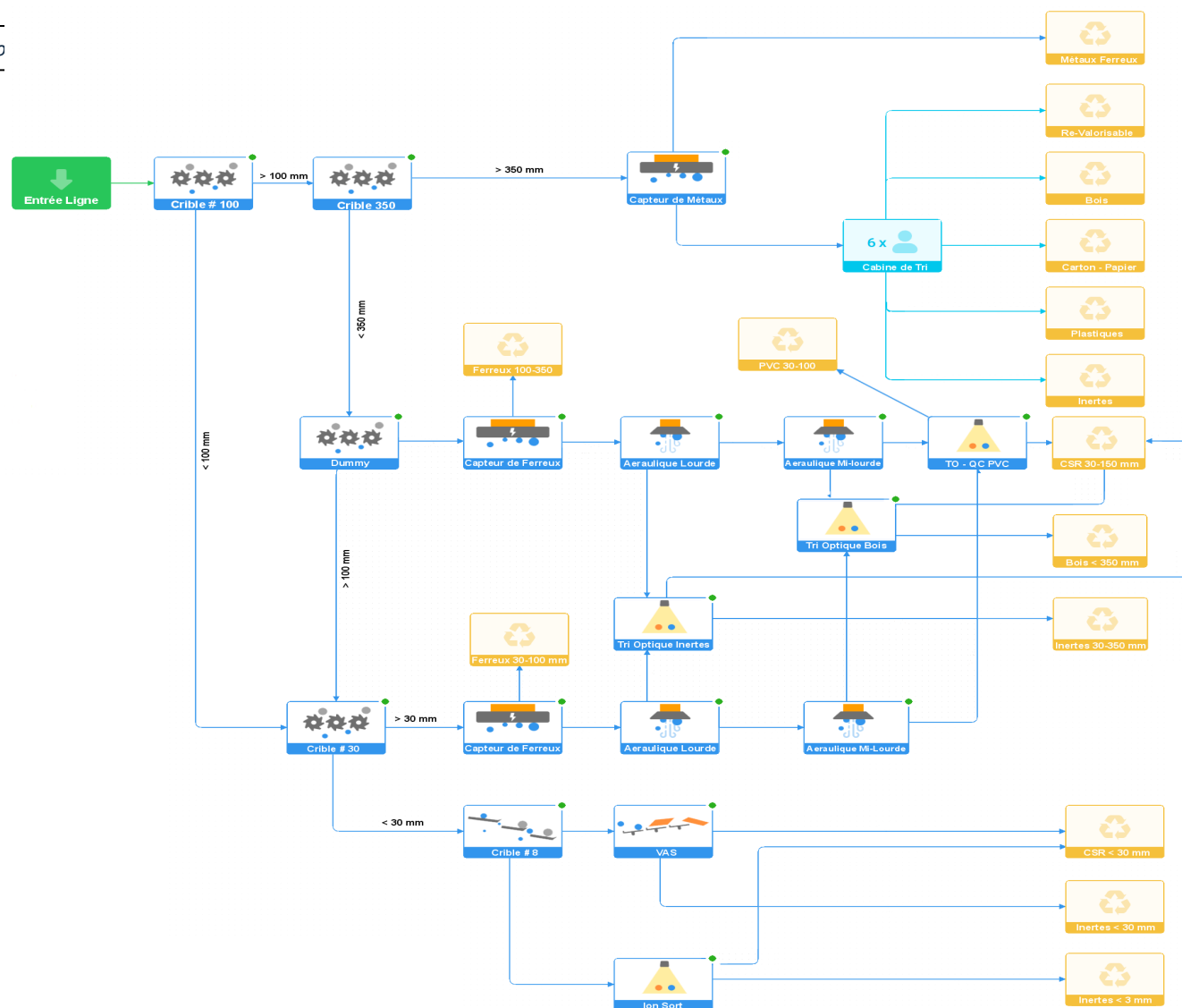
Figure 13 : Principe de séparation
