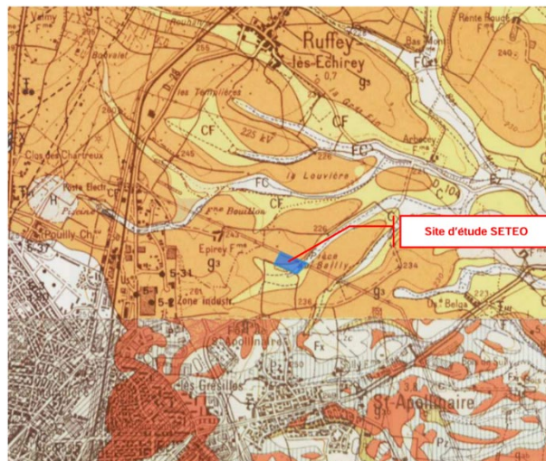
Figure 23 : Carte géologique échelle 1/25000 (source : BRGM)
