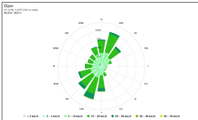
Figure 22 : Rose des vents à Dijon (MétéoBlue)
