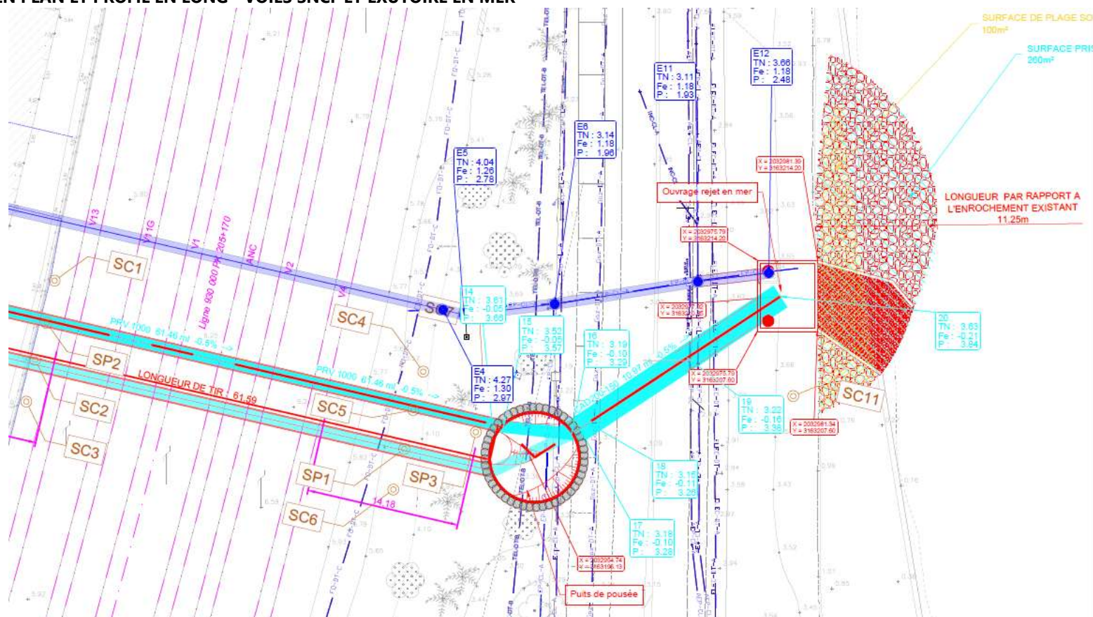
FIGURE 4 : VUE EN PLAN ET PROFIL EN LONG - VOIES SNCF ET EXUTOIRE EN MER
