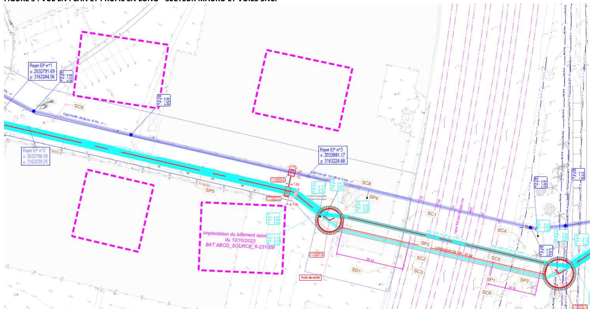
FIGURE 3 : VUE EN PLAN ET PROFIL EN LONG - SECTEUR MAURO ET VOIES SNCF
