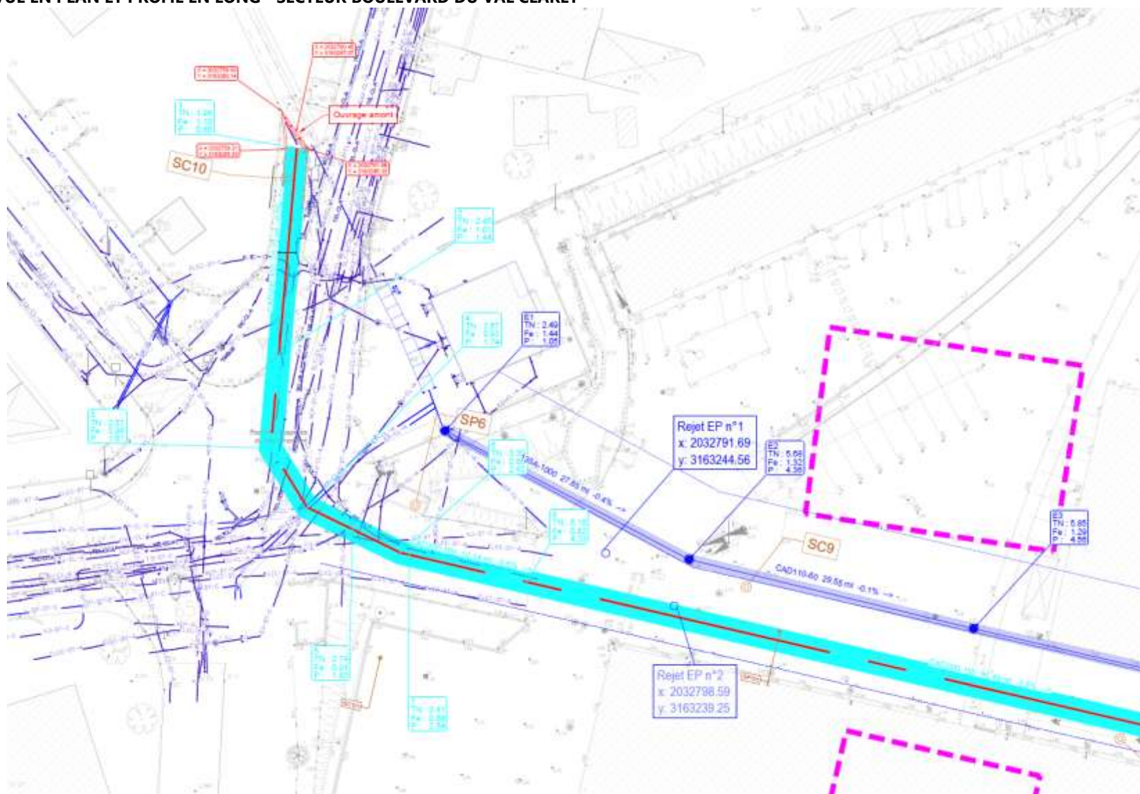
FIGURE 2 : VUE EN PLAN ET PROFIL EN LONG - SECTEUR BOULEVARD DU VAL CLARET
