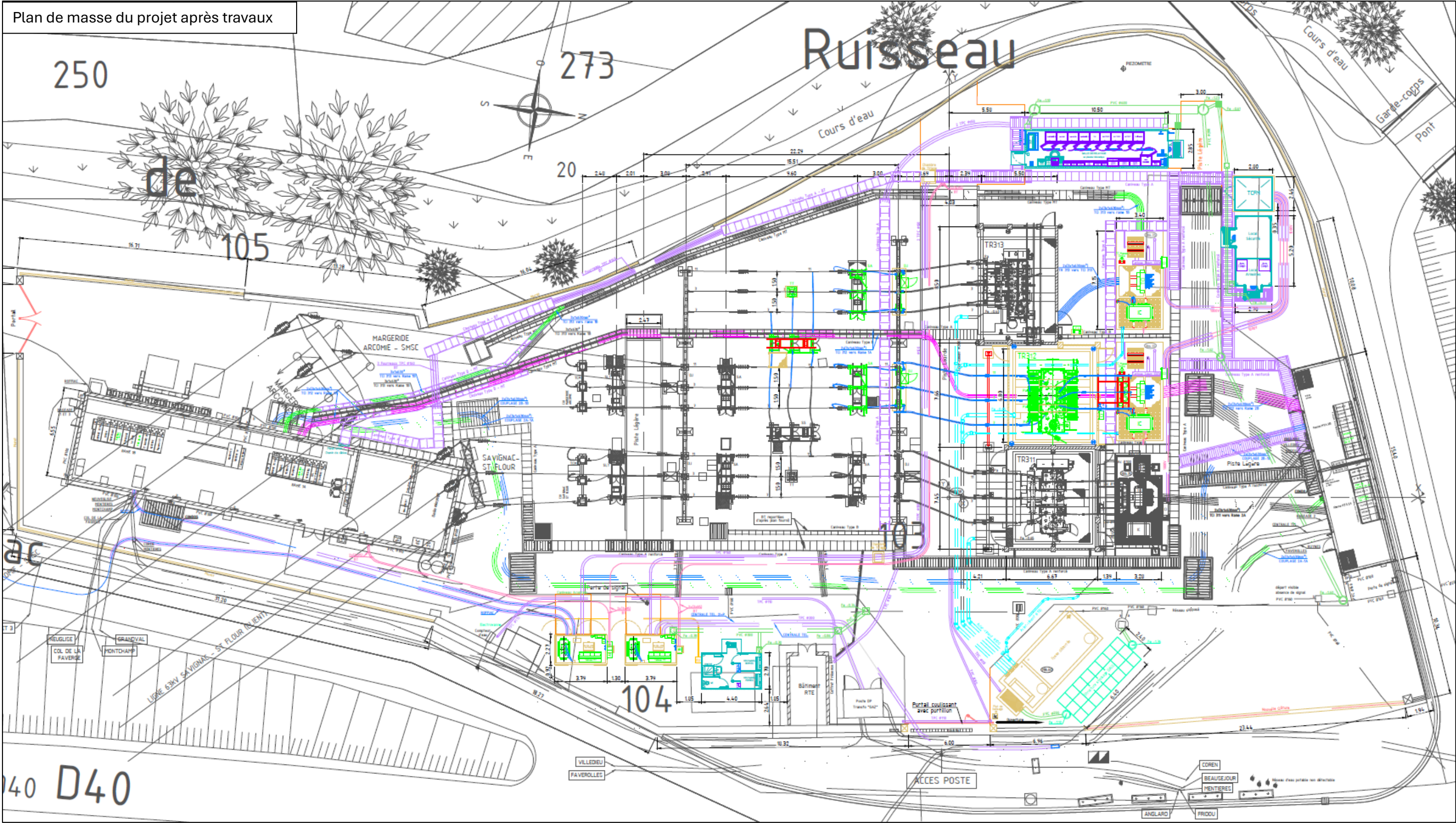
Annexe 5 : Plan du projet
