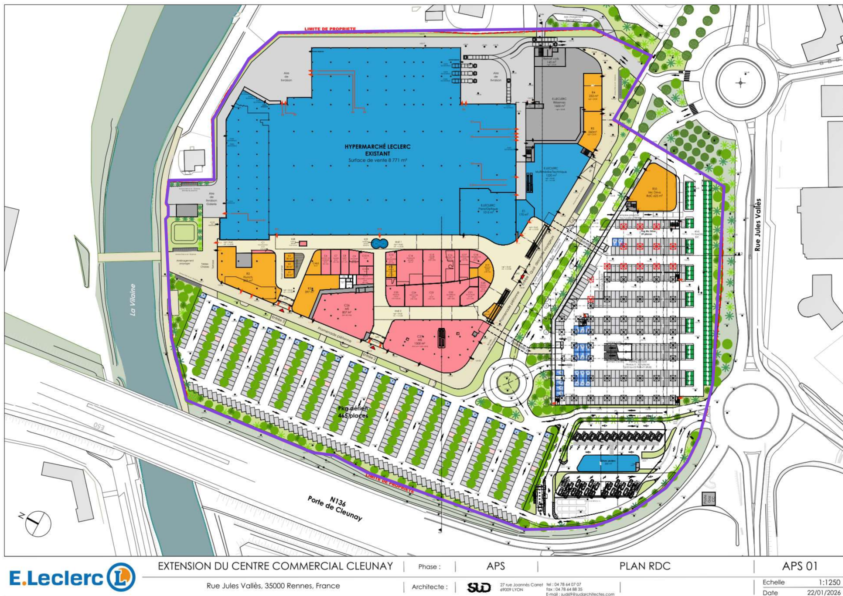
Plan du rez-de-chaussée du projet d'extension du centre commercial Cleunay, SUD Architectes, 2026
