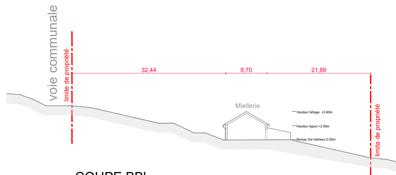
COUPE BB'
