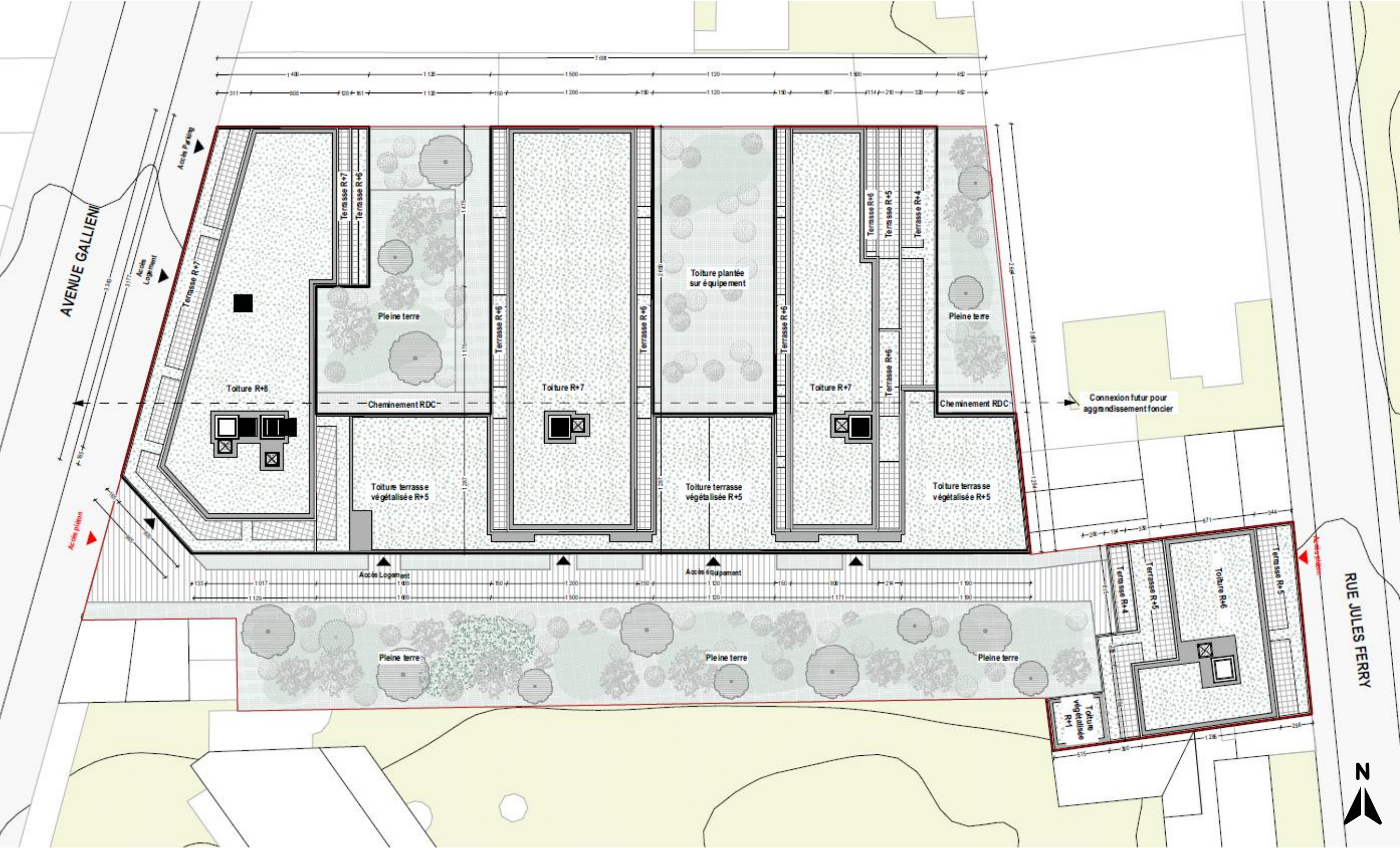
Plan de masse du projet – Architectures Singulières, Octobre 2025
