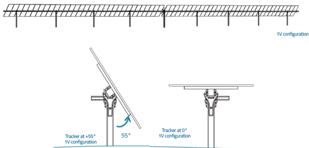
Figure 1 : Schéma d'une table de modules
