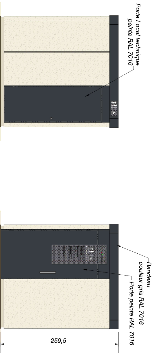
Façade Sud-Ouest
