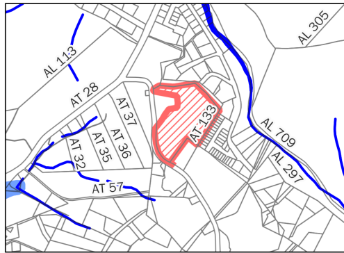
Zonage de faille:
