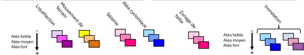
Cartes des aléas naturel à l'échelle de la parcelle
