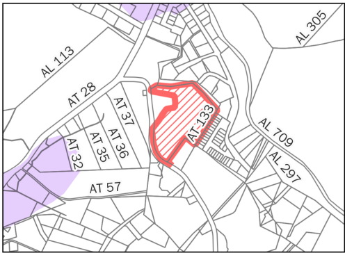
Aléa mouvement de terrain:
