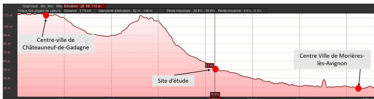
Figure 13 : Analyse du profil altimétrique entre le centre-ville de Châteauneuf-de-Gadagne, le site d'étude et le centre-ville de Morières-lès-Avignon – Source : Google Earth Pro
