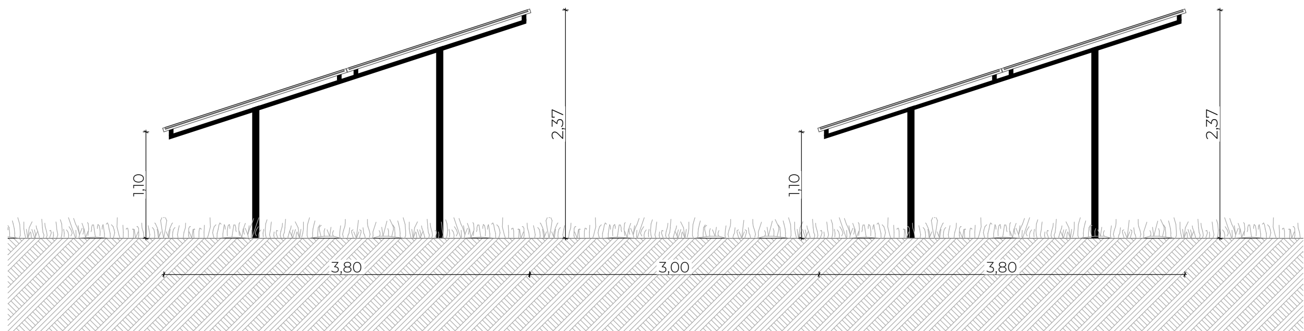
DP Annexe - Distance minimale entre deux rangées
