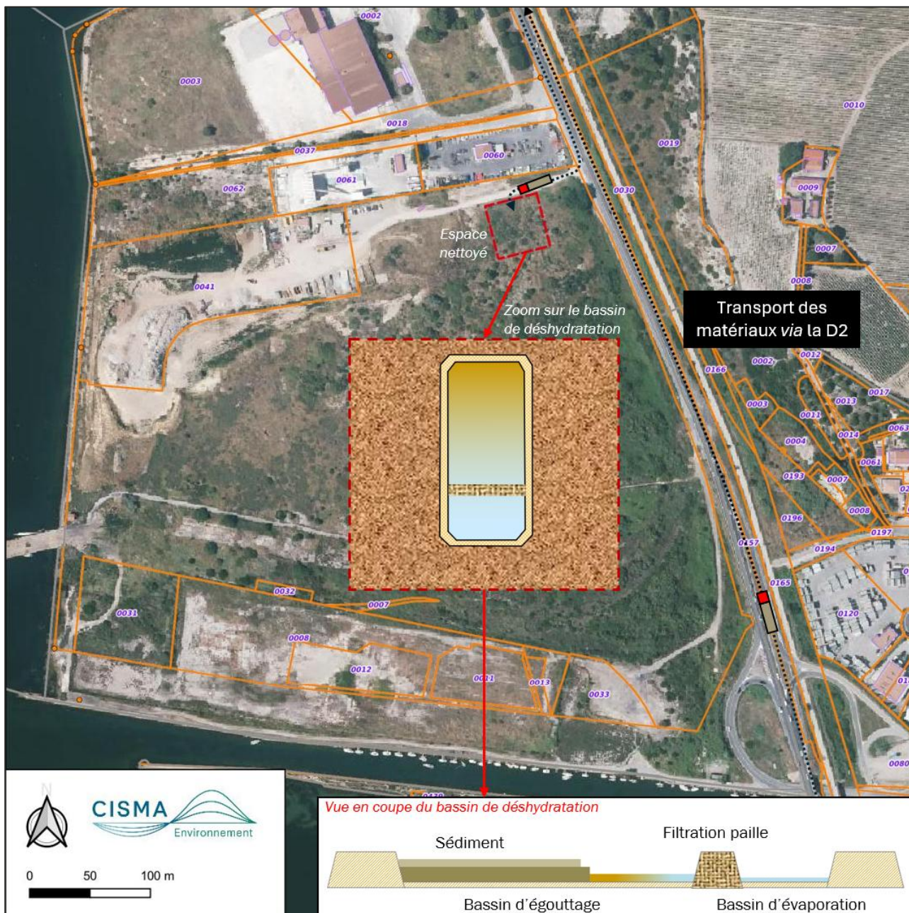
Schéma de principe des opérations de déshydratation des matériaux sur la parcelle DK0044
